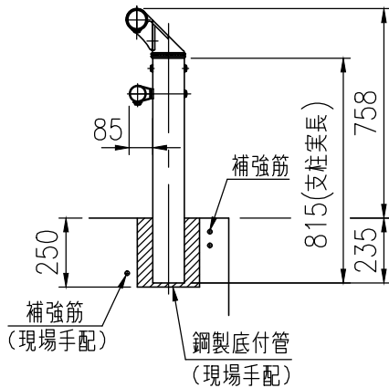
上段ビームパイプ詳細図 (1/10)
