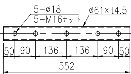
上段インナースリーブ詳細図 (1/10)
