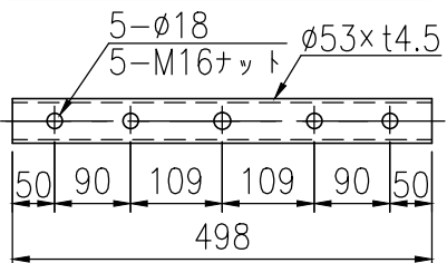
下段インナースリーブ詳細図 (1/10)
