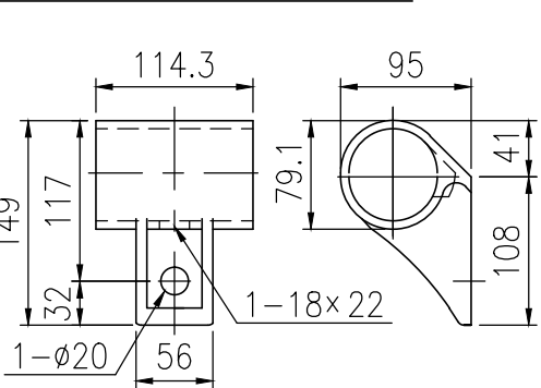
上段ビームコネクター詳細図 (1/6)
