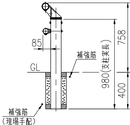
上段インナースリーブ詳細図 (1/10)
