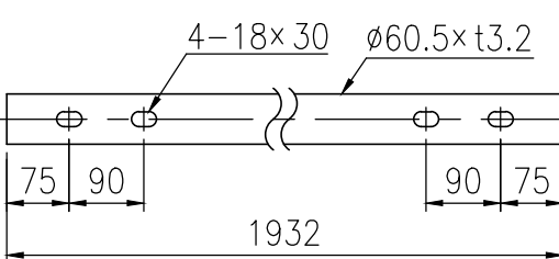
下段ビームパイプ詳細図 (1/10)
