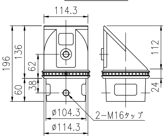
キャップ詳細図 (1/6)
