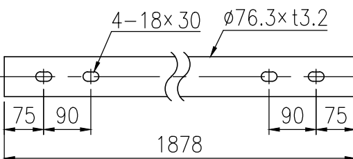
上段ビームパイプ詳細図 (1/10)
