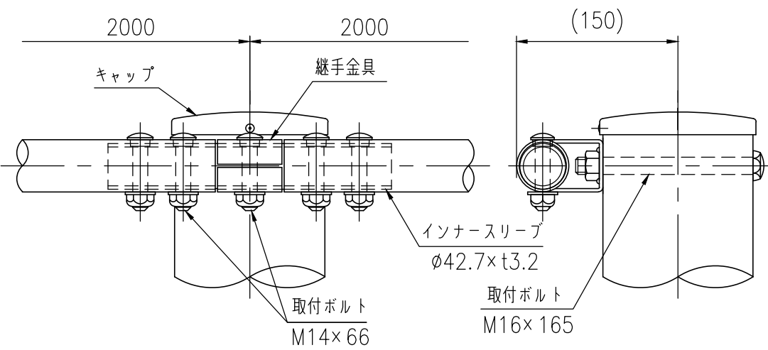
中間部詳細図 (1/5)
