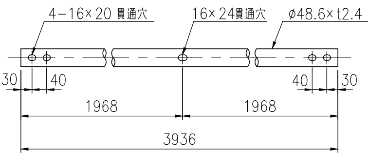
ビームパイプ詳細図 (1/10)
