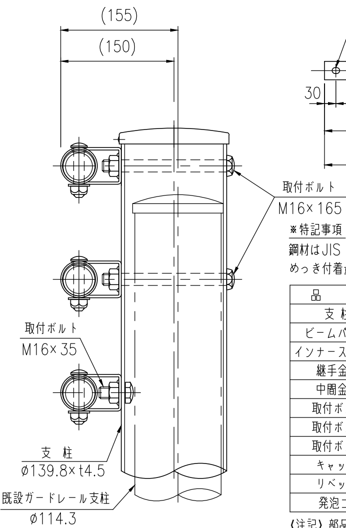
支柱詳細図 (1/5)
