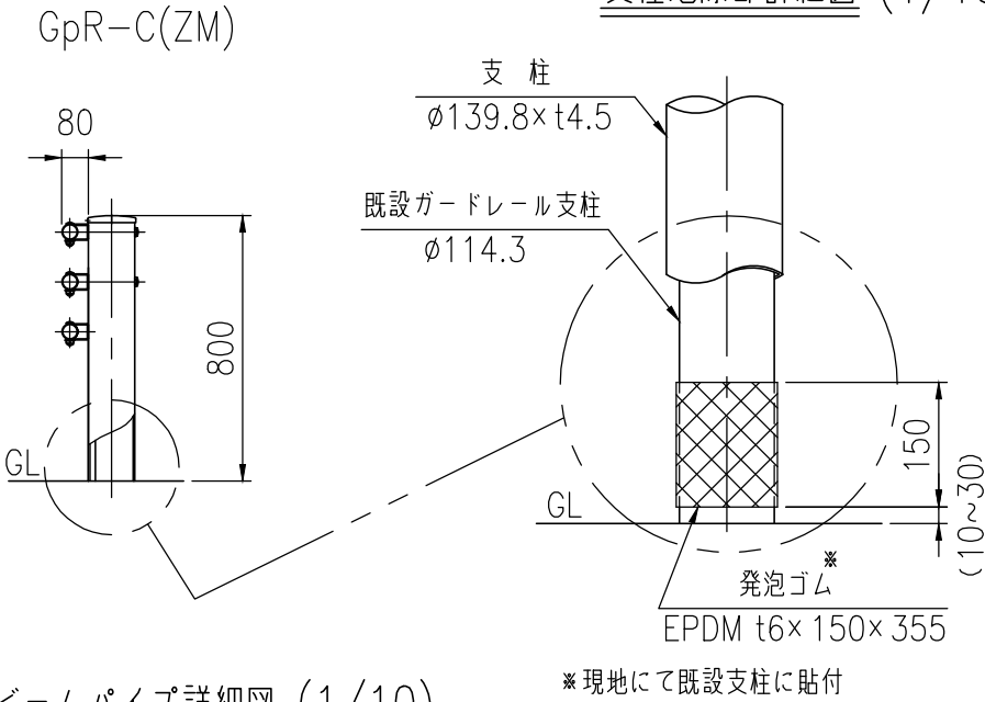
ビームパイプ詳細図 (1/10)
