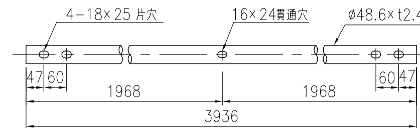
ビームパイプ詳細図 (1/10)
