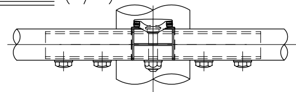
中間部詳細図 (1/6)
