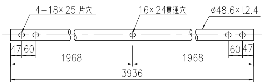
ビームパイプ詳細図 (1/10)
