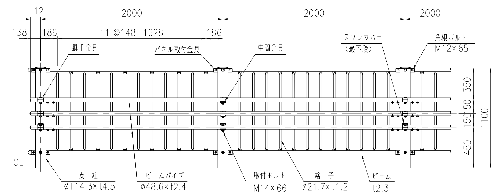
設置図 (1/25)
