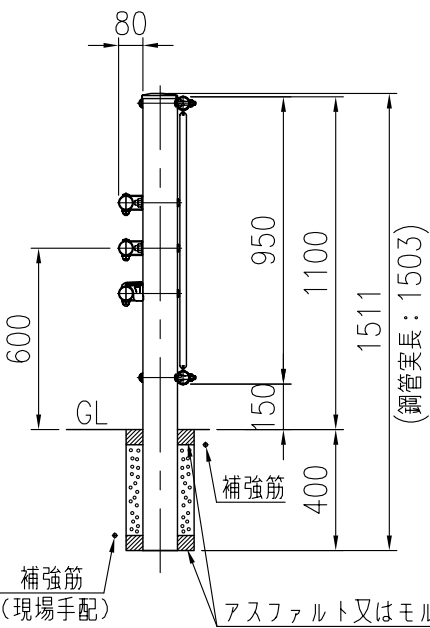
GpLXT-C-2B
