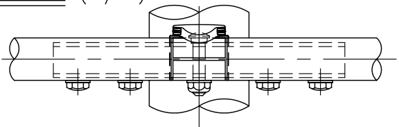
中間部詳細図 (1/6)
