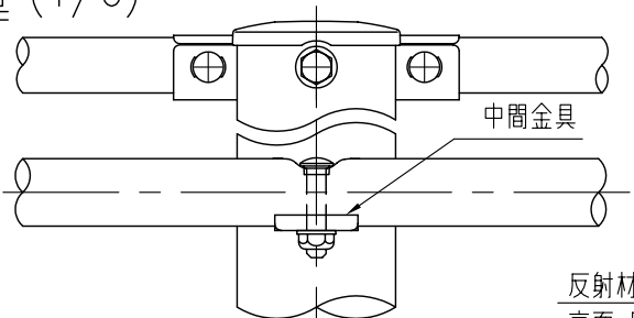
中間部最下段詳細図 (1/6)
