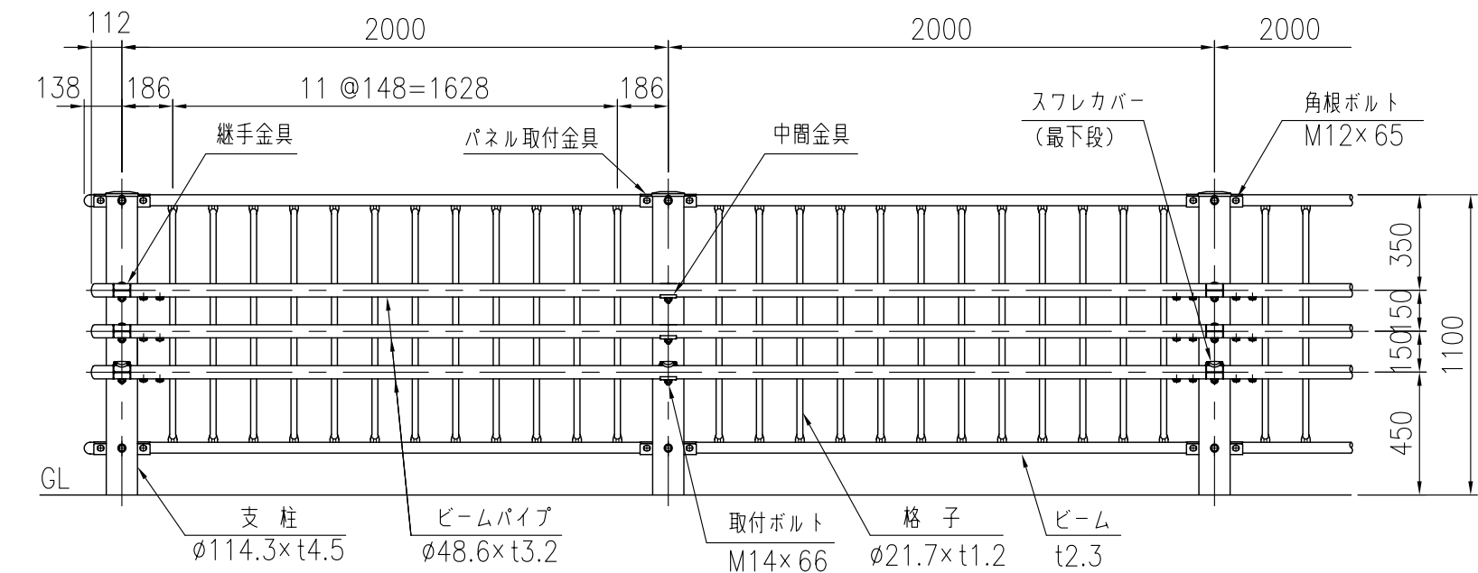
設置図 (1/25)
