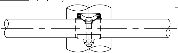
中間部最下段詳細図 (1/6)
