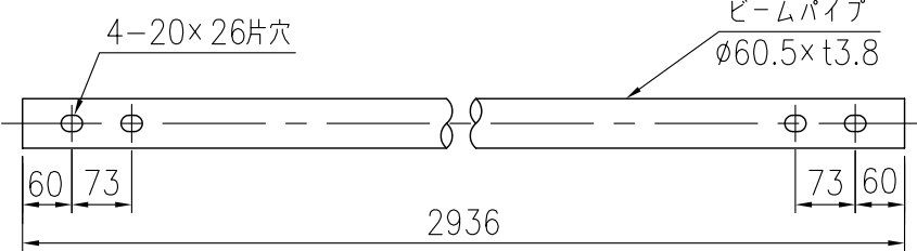
ビームパイプ詳細図 (1/10)
