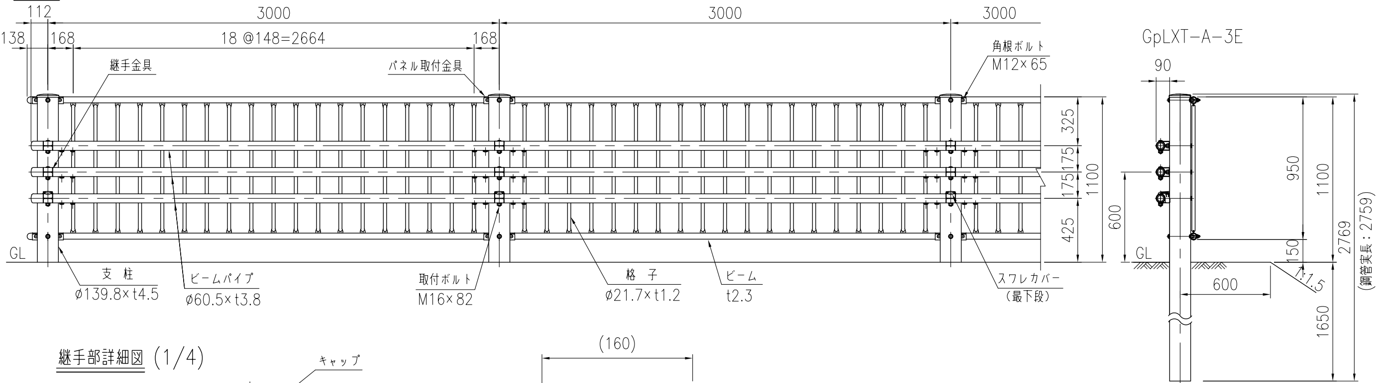
設置図 (1/25)
