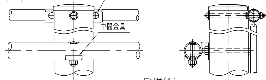
中間部最下段詳細図 (1/8)
