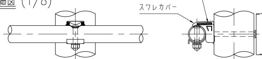
中間部最下段詳細図 (1/8)
