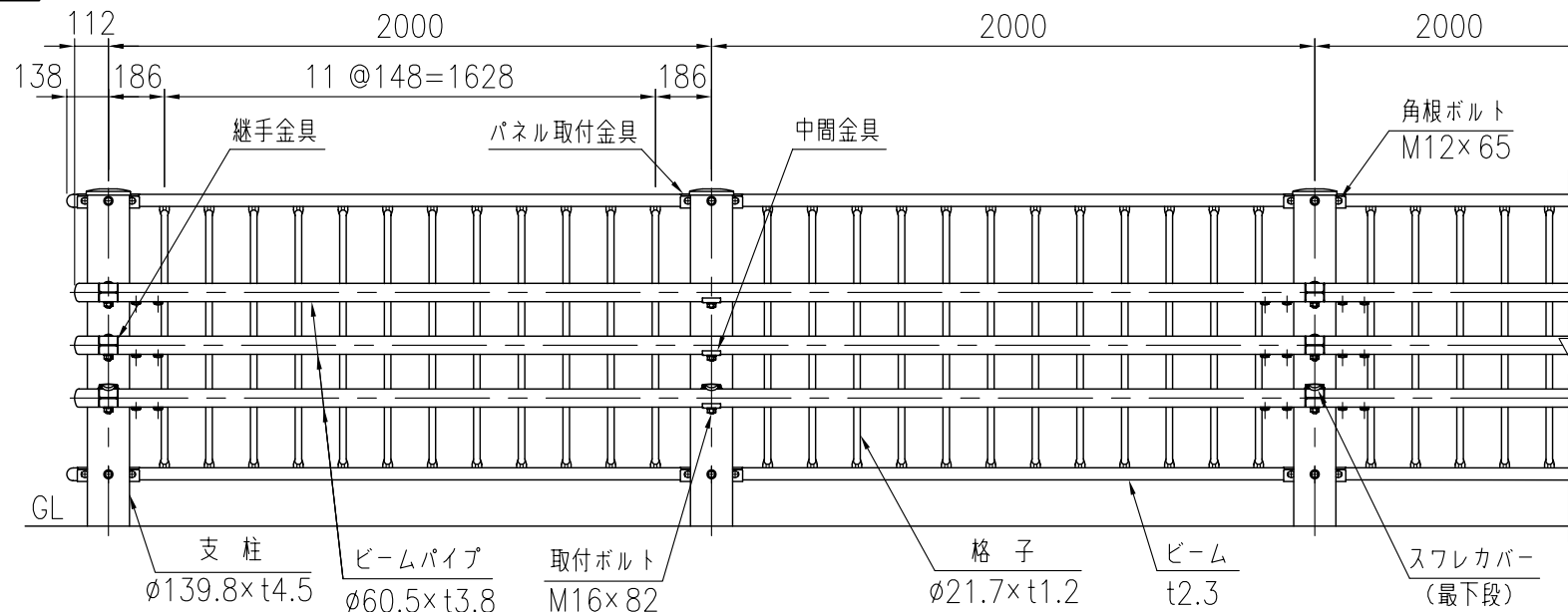
設置図 (1/25)
