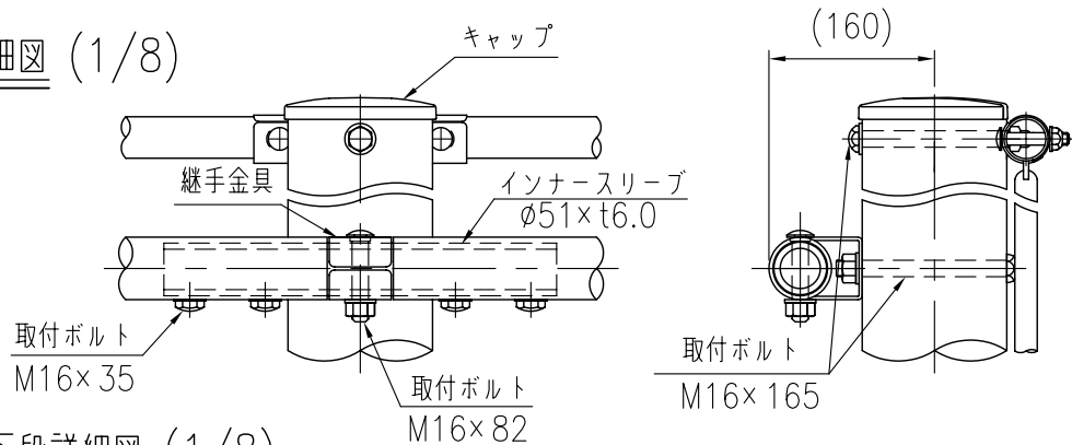
継手部最下段詳細図 (1/8)
