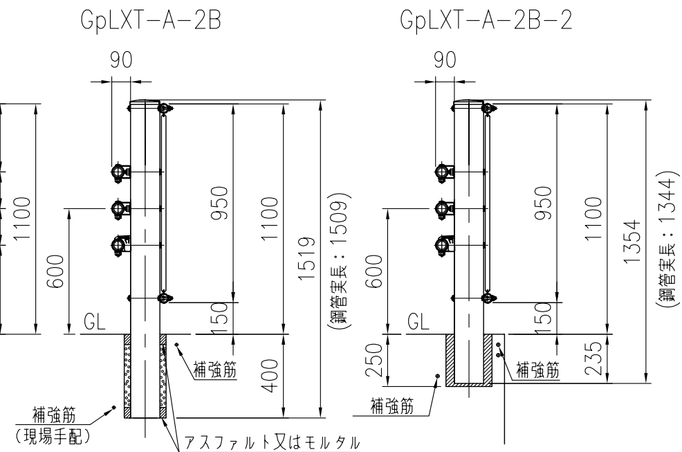
ビームパイプ詳細図 (1/10)
