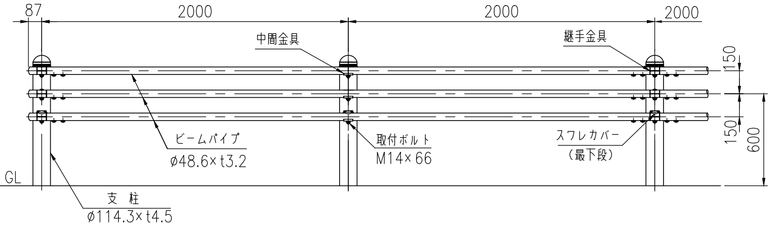
設置図 (1/25)
