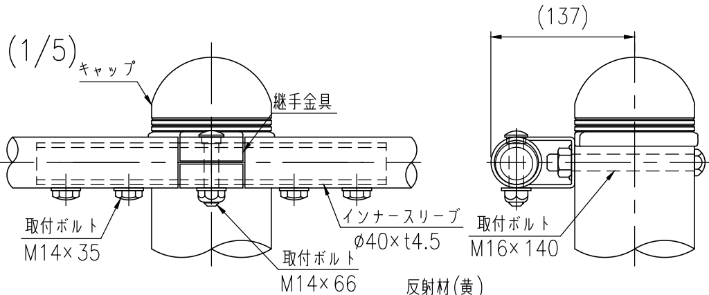
継手部最下段詳細図 (1/5)
