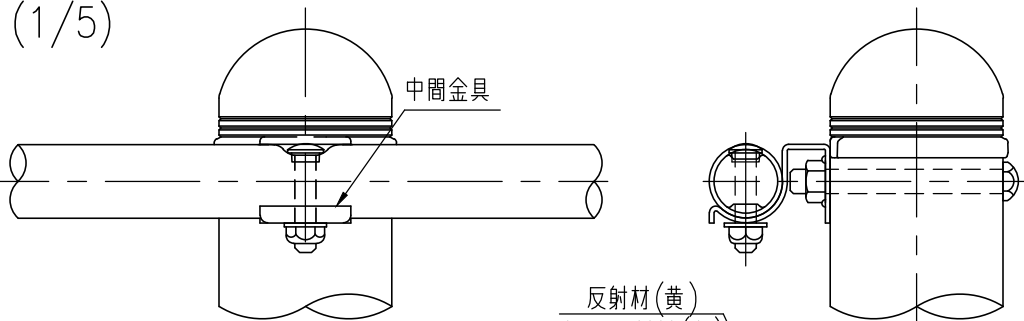
中間部最下段詳細図 (1/5)
