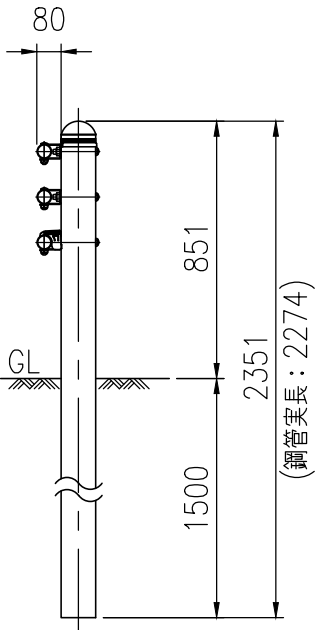
GpLM-Bp-2E (ZM) (歩車道境界用)
