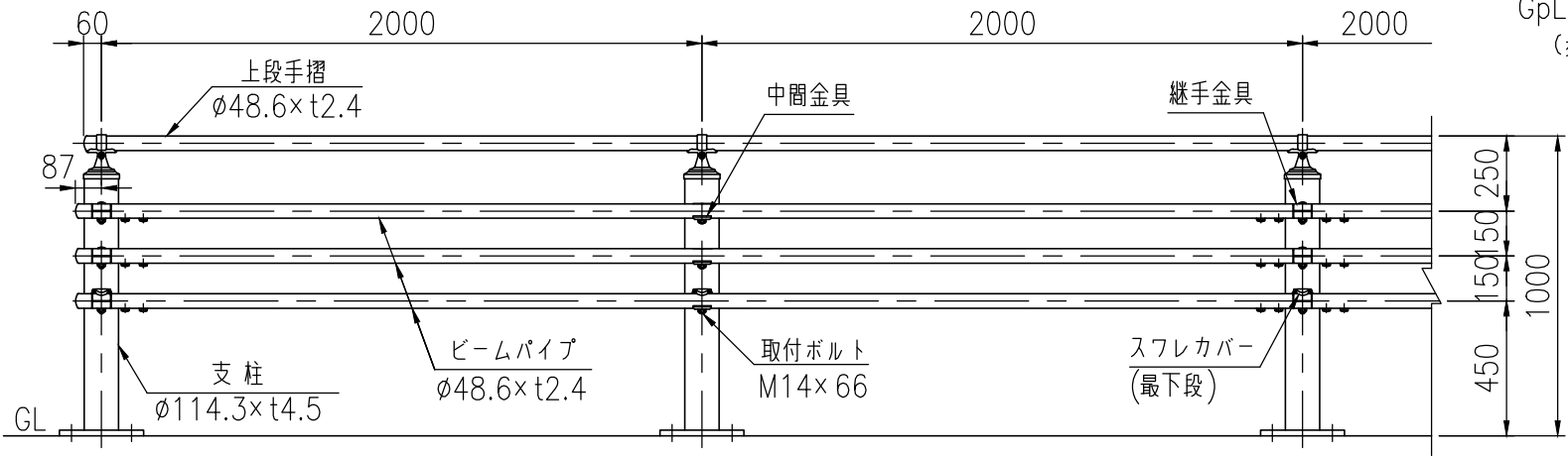
設置図 (1/25)
