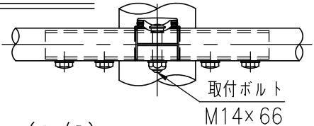
中間部詳細図 (1/8)
