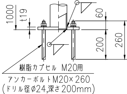
ベースプレート詳細図 (1/15)
