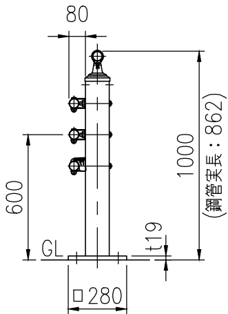
ビームパイプ詳細図 (1/10)
