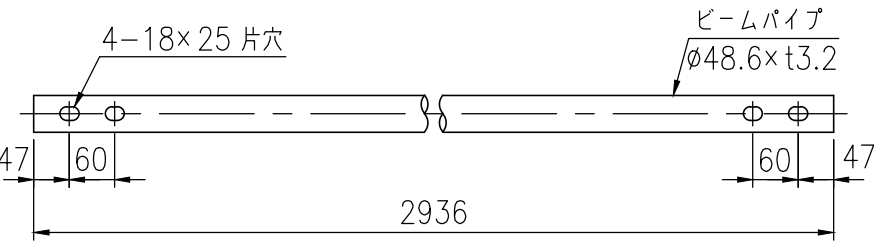
ビームパイプ詳細図 (1/10)
