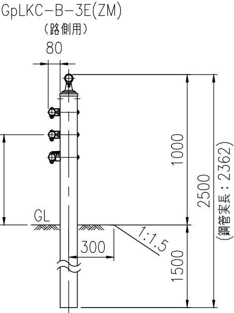
ビームパイプ詳細図 (1/10)
