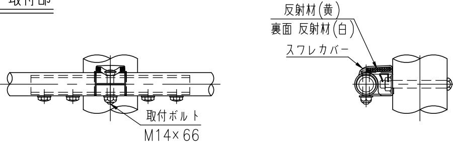
スフレカバー取付部
