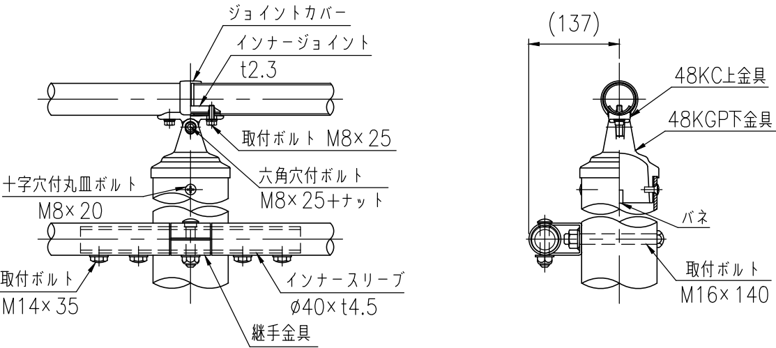
継手部詳細図 (1/8)
