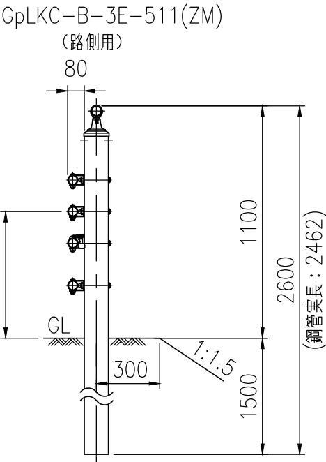
ビームパイプ詳細図 (1/10)
