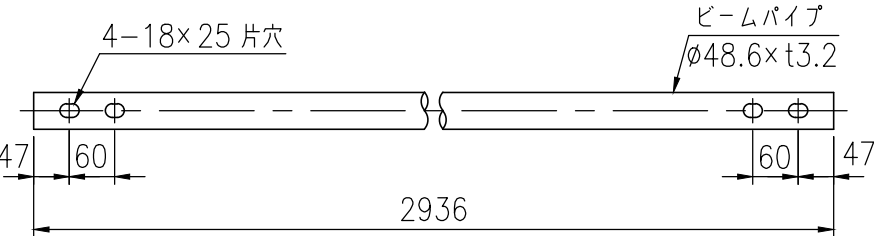
ビームパイプ詳細図 (1/10)
