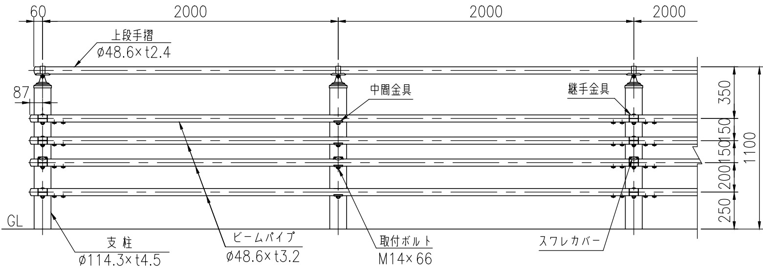
設置図 (1/25)
