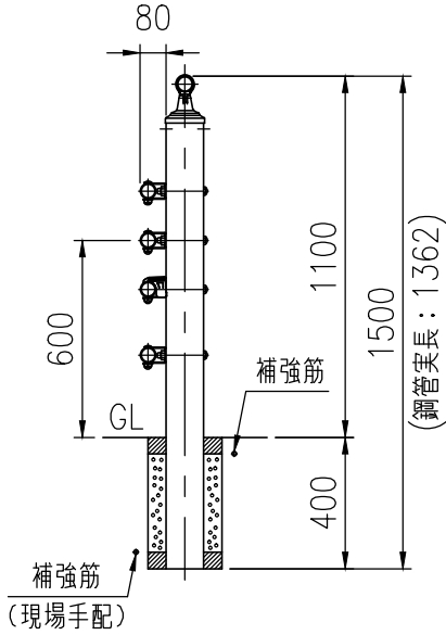
ビームパイプ詳細図 (1/10)
