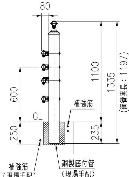
GpLKC-B-2B-2-511(ZM) (路側用)
