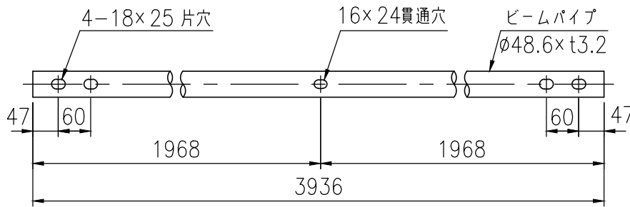
梁パイプ詳細図 (1/10)
