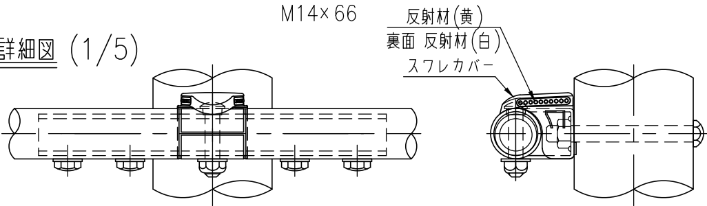
中間部詳細図 (1/5)
