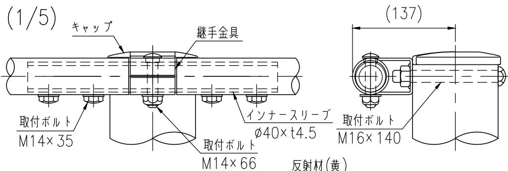
継手部最下段詳細図 (1/5)
