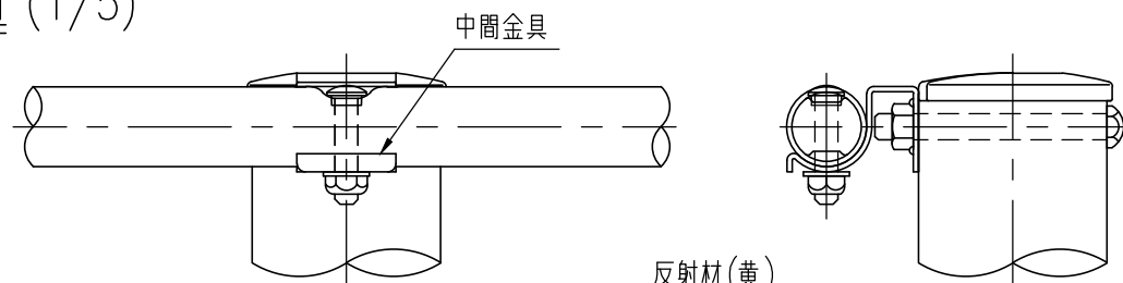
中間部最下段詳細図 (1/5)
