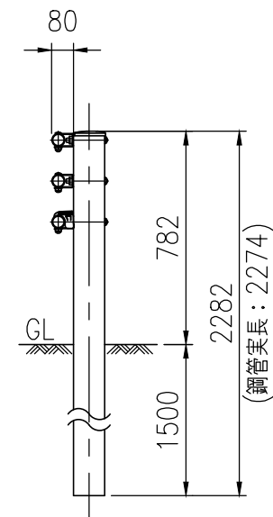
ビームパイプ詳細図 (1/10)
