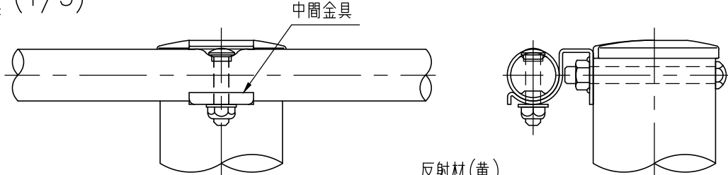
中間部最下段詳細図 (1/5)
