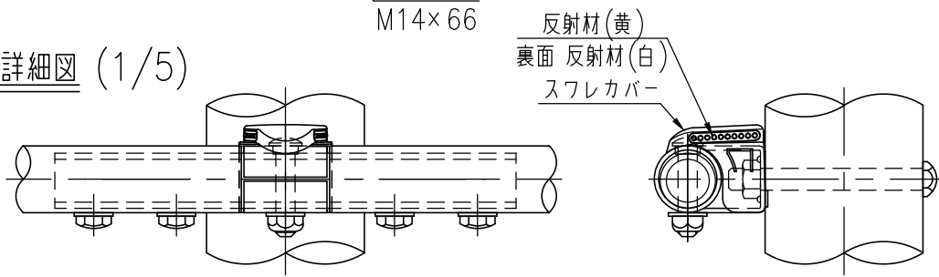
中間部詳細図 (1/5)
