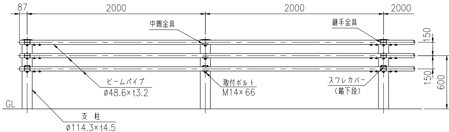
設置図 (1/25)
