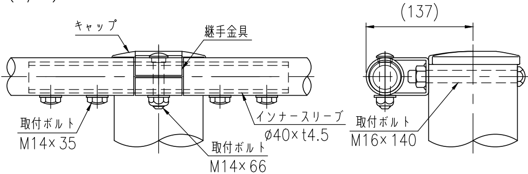
継手部詳細図 (1/5)
