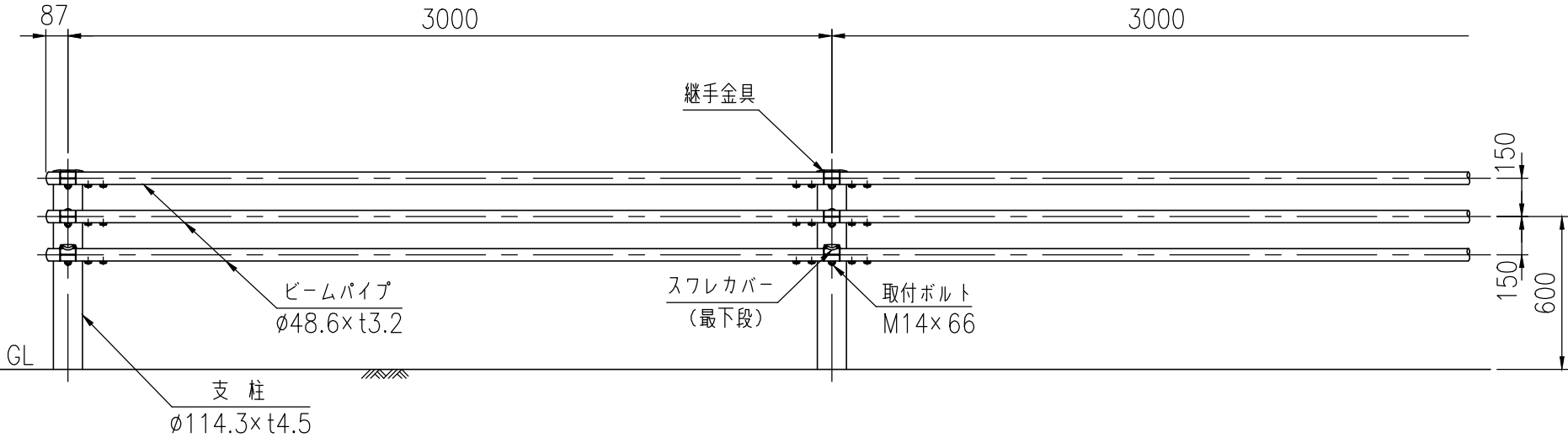
設置図 (1/25)
