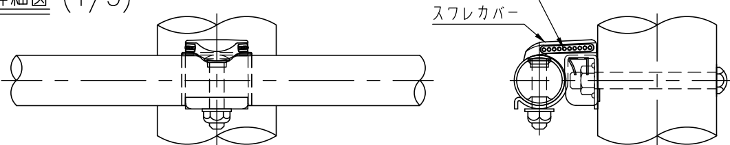
中間部最下段詳細図 (1/5)
