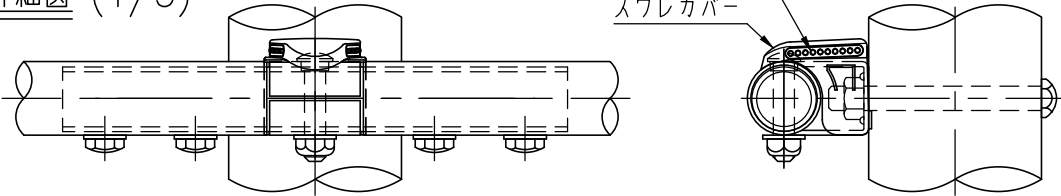
継手部最下段詳細図 (1/5)
