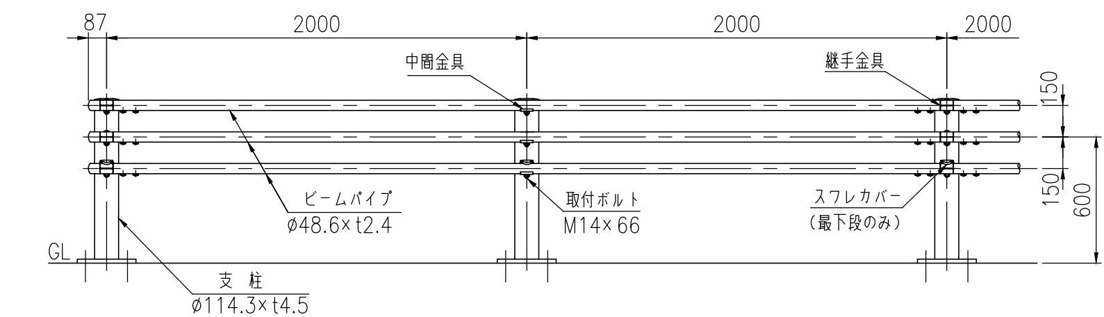
設置図 (1/25)
