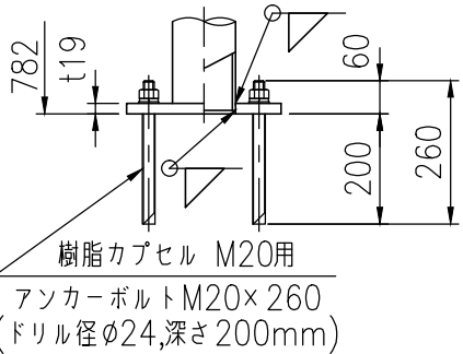
ベースプレート詳細図 (1/15)
