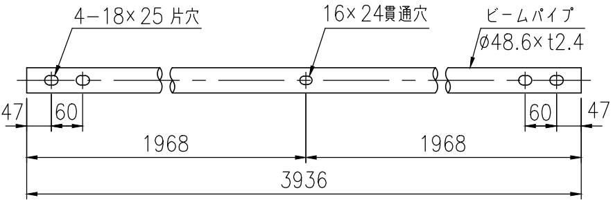
光束パイプ詳細図 (1/10)
