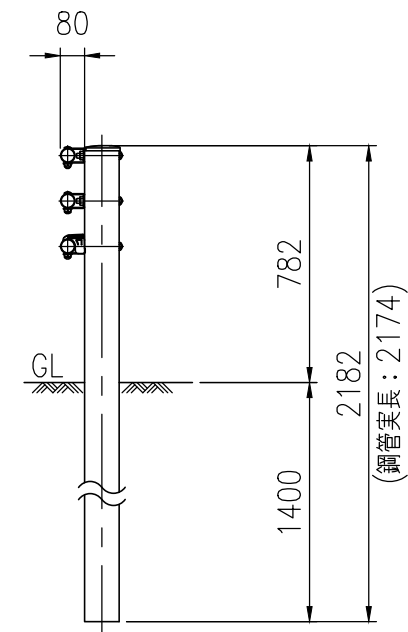
ビームパイプ詳細図 (1/10)
