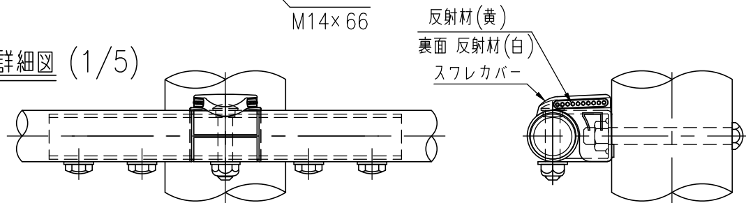
中間部詳細図 (1/5)
