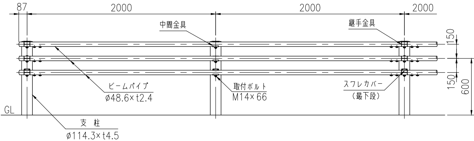
設置図 (1/25)
