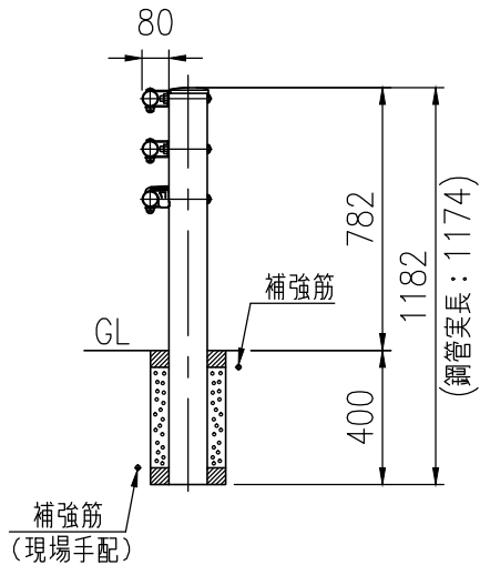
GpL-Cp-2B(ZM)・GpL-C-2B(ZM) (歩車道境界用) (路側用)
