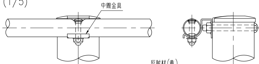
中間部最下段詳細図 (1/5)
