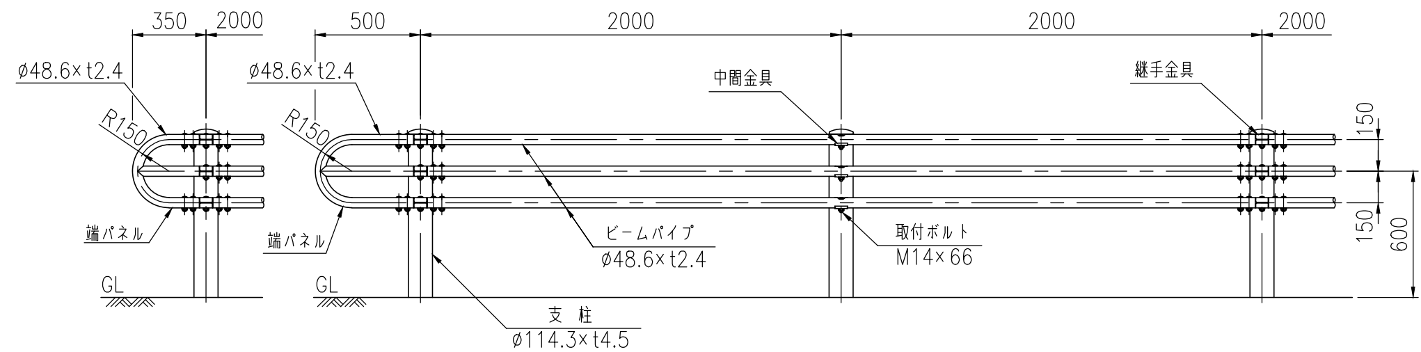
設置図 (1/25)
