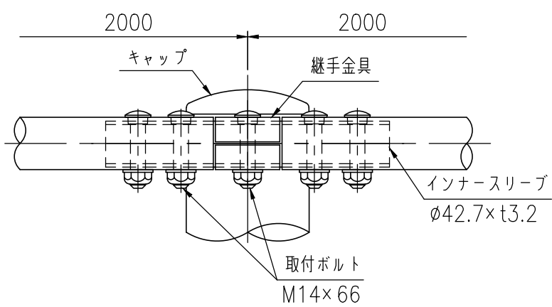
中間部詳細図 (1/5)
