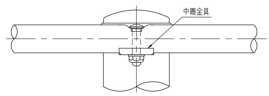
中間部詳細図 (1/4)
