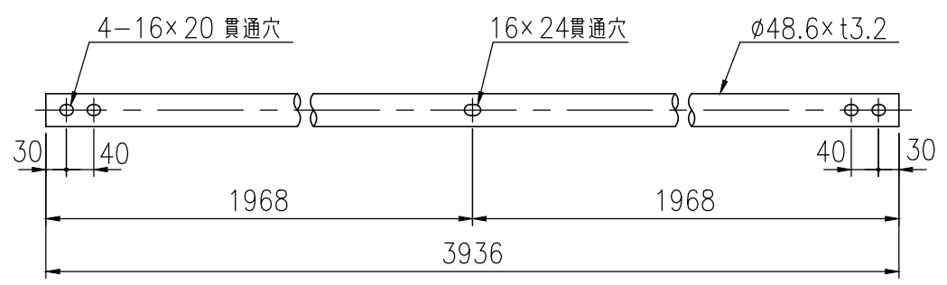
ビームパイプ詳細図 (1/10)
