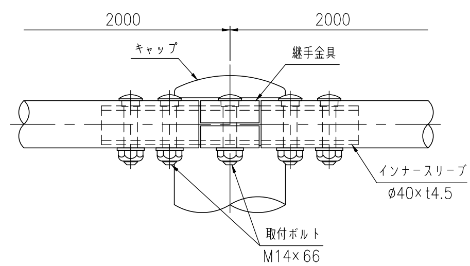
中間部詳細図 (1/4)
