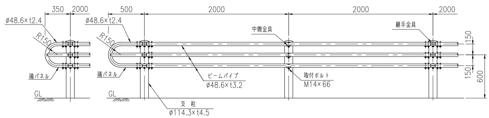
設置図 (1/25)
