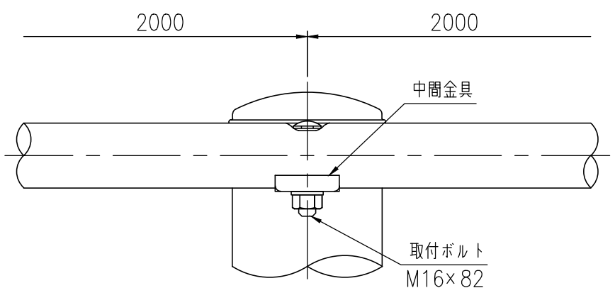
中間部詳細図 (1/5)
