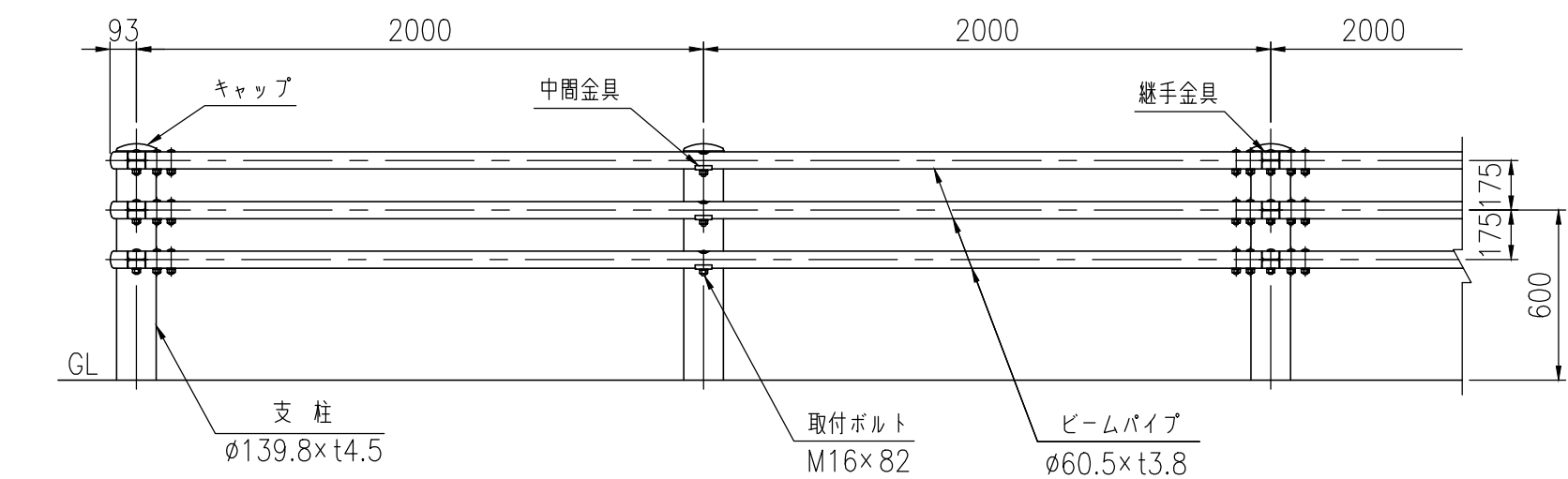
設置図 (1/25)
