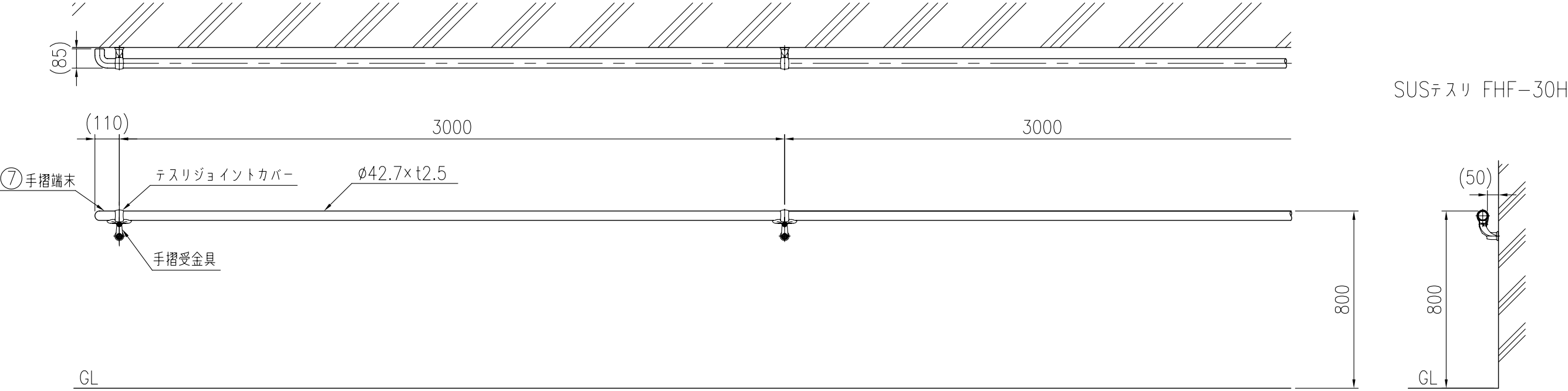
設置図 (1/20)
