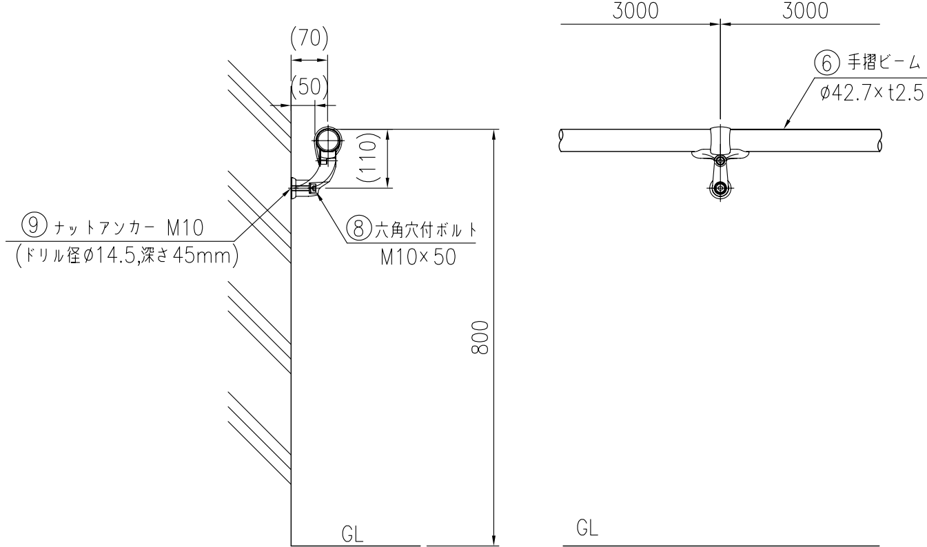
取付図 (1/10)
