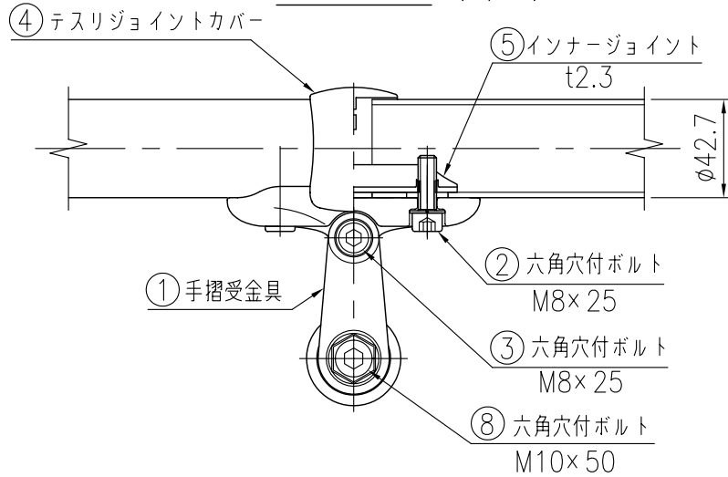
取付部詳細図 (1/3)
