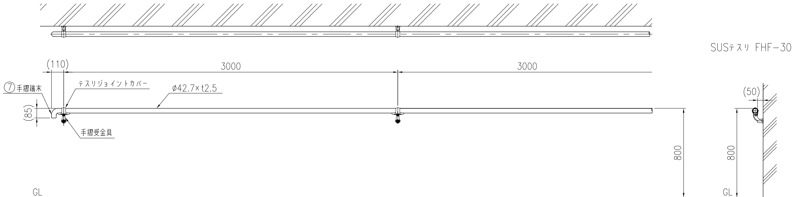
設置図 (1/20)
