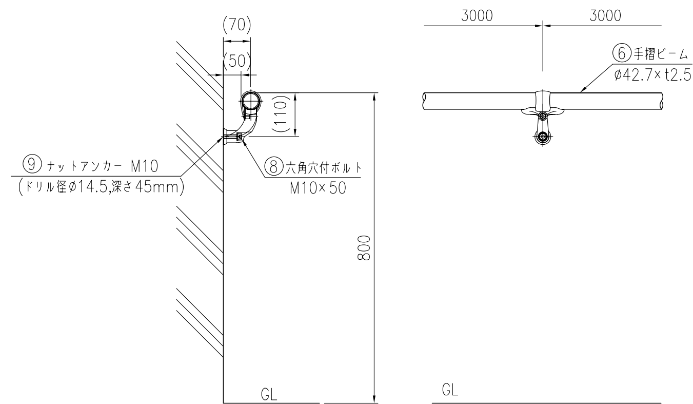
取付図 (1/10)
