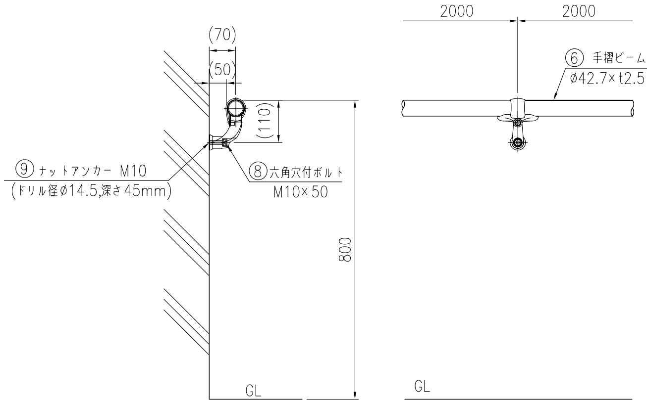
取付図 (1/10)
