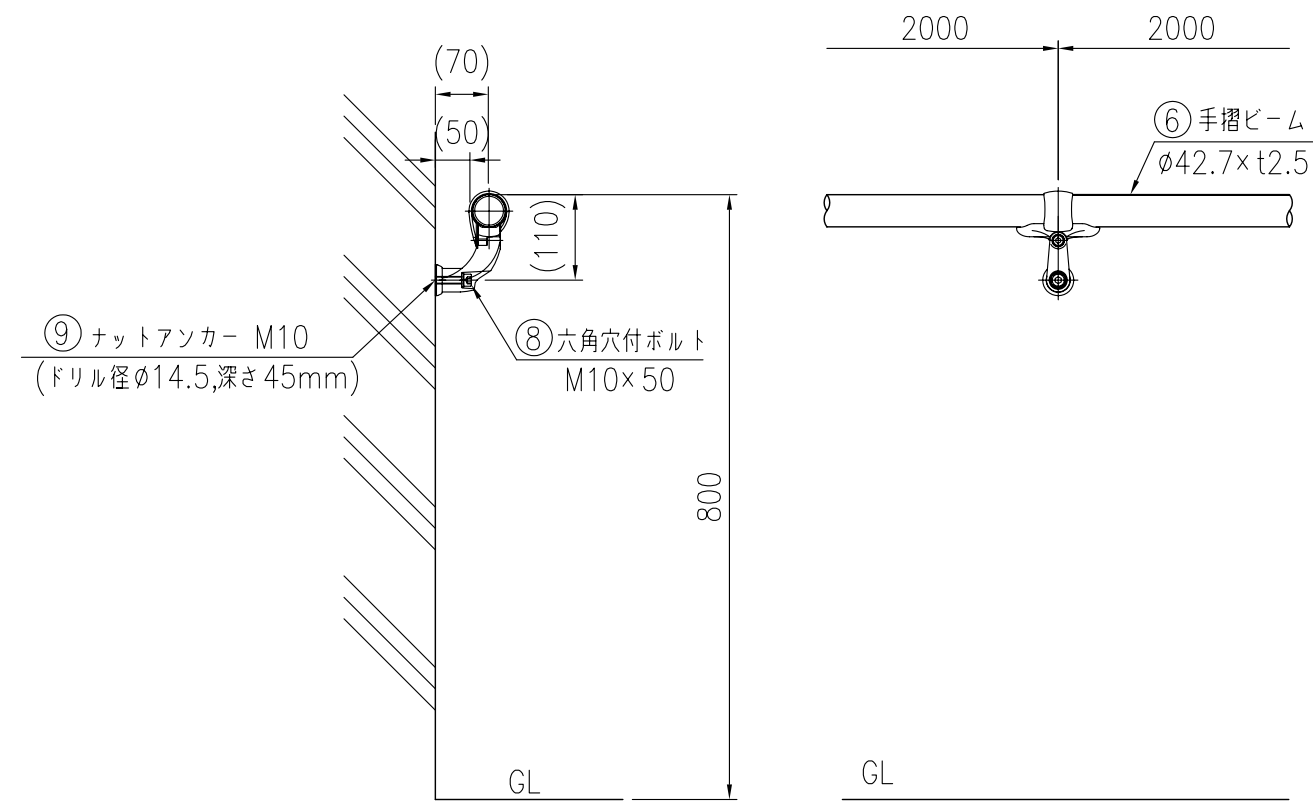
取付図 (1/10)
