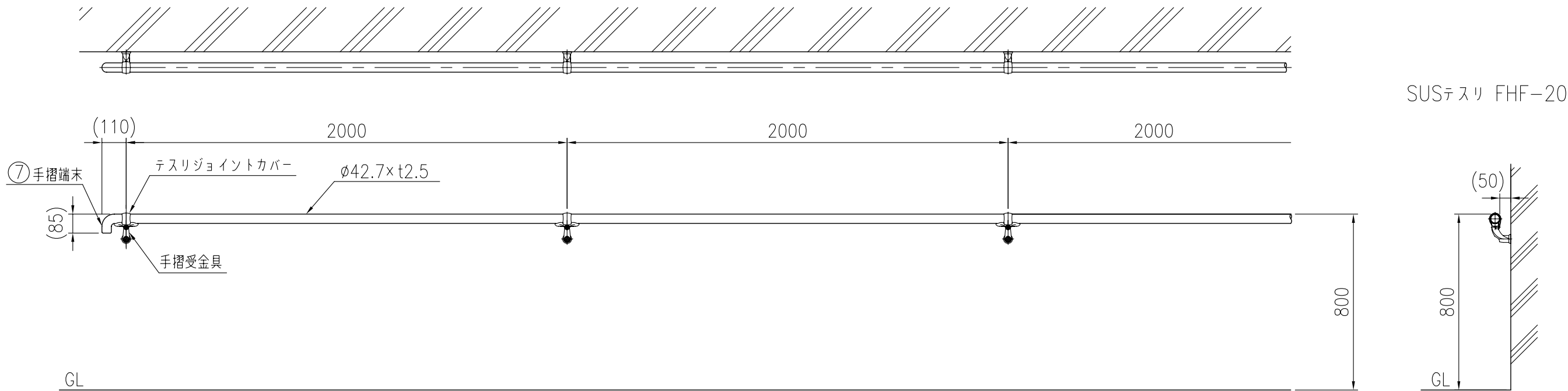
設置図 (1/20)
