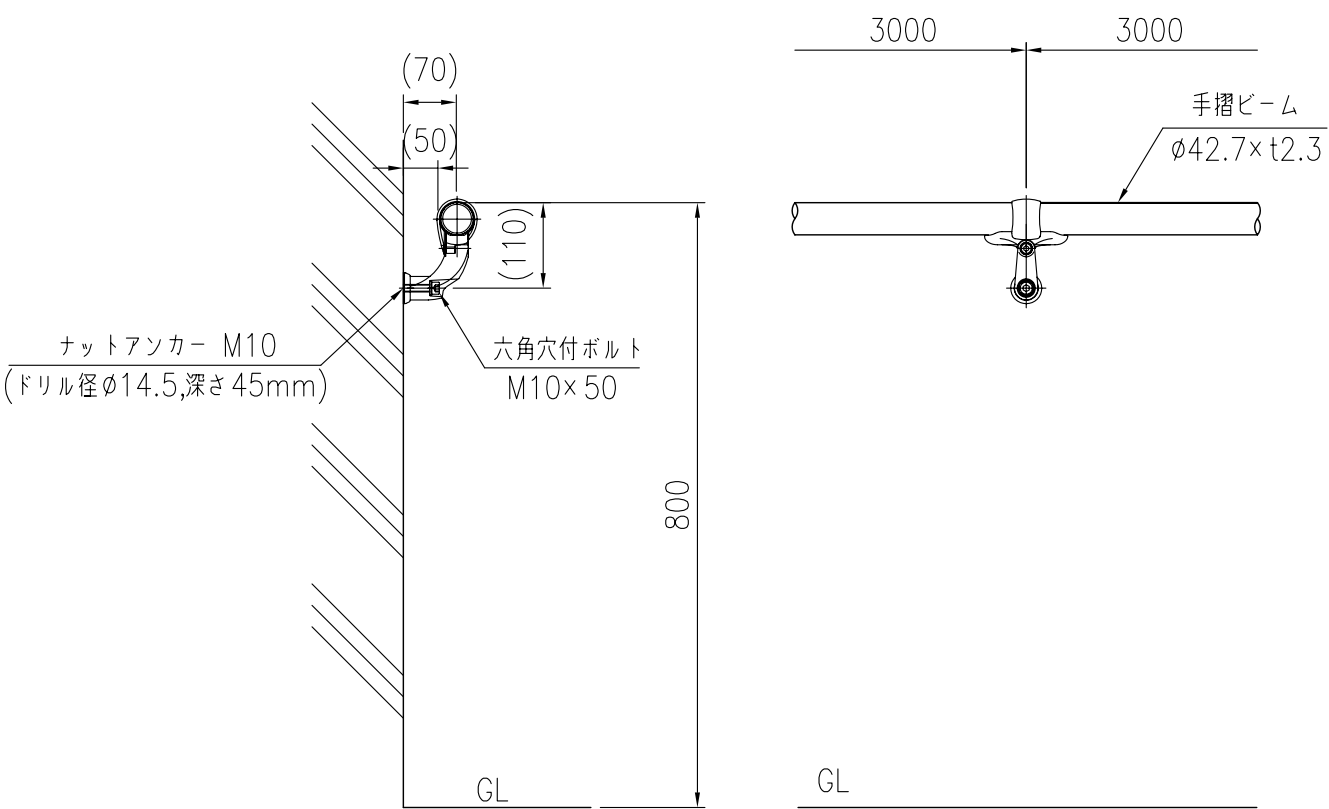
取付図 (1/10)
