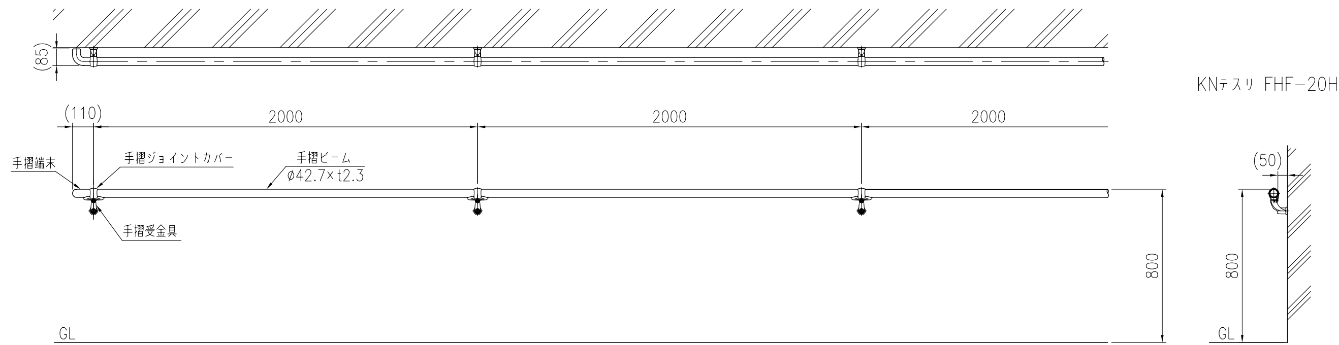
設置図 (1/20)
