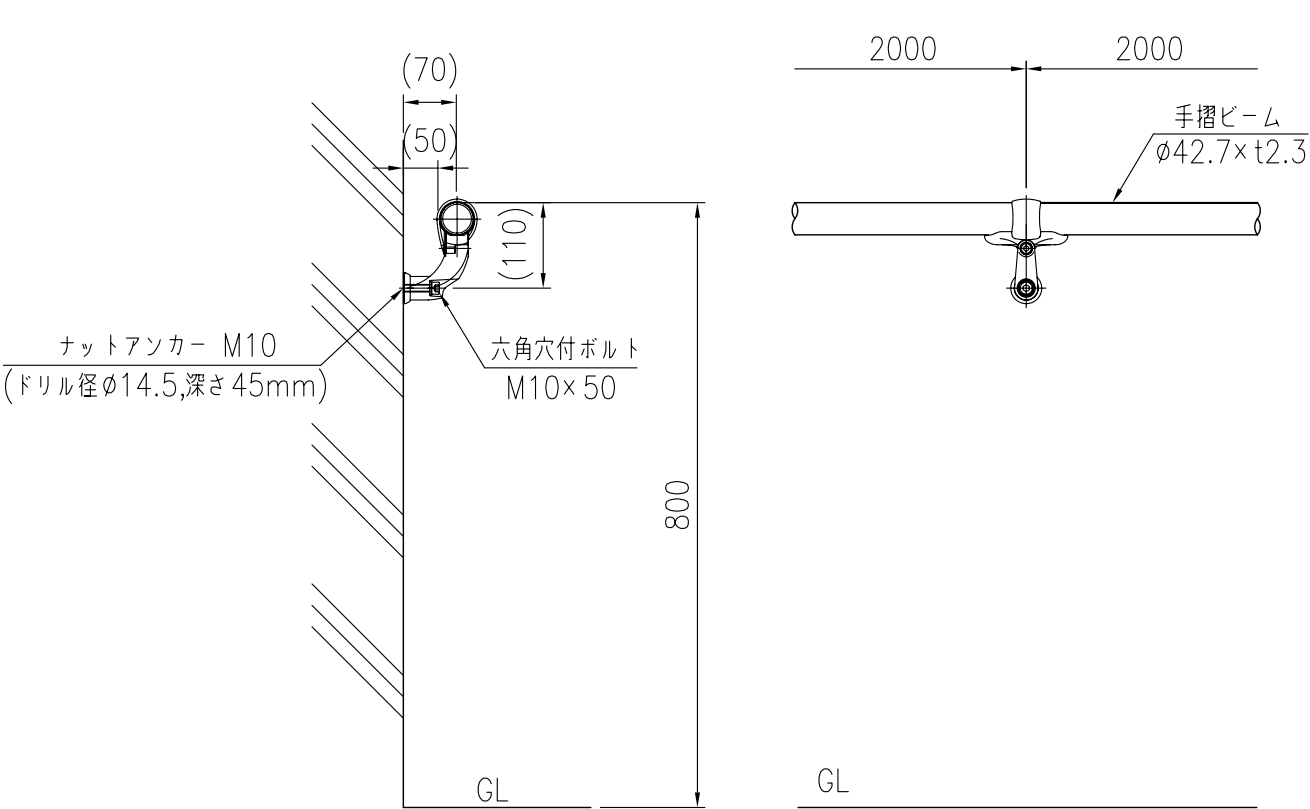
取付図 (1/10)
