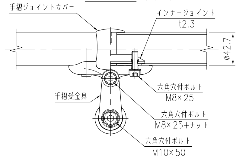
取付部詳細図 (1/3)
