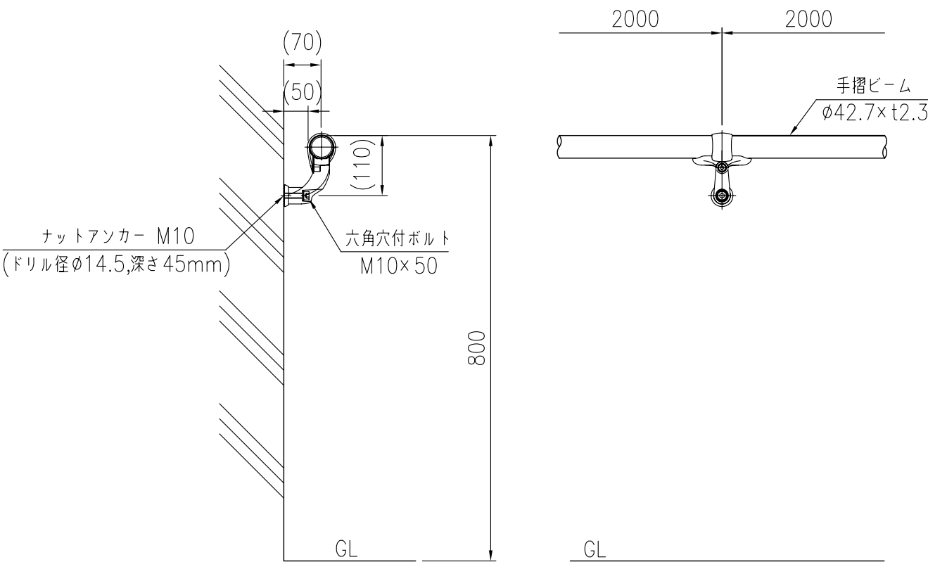
取付図 (1/10)
