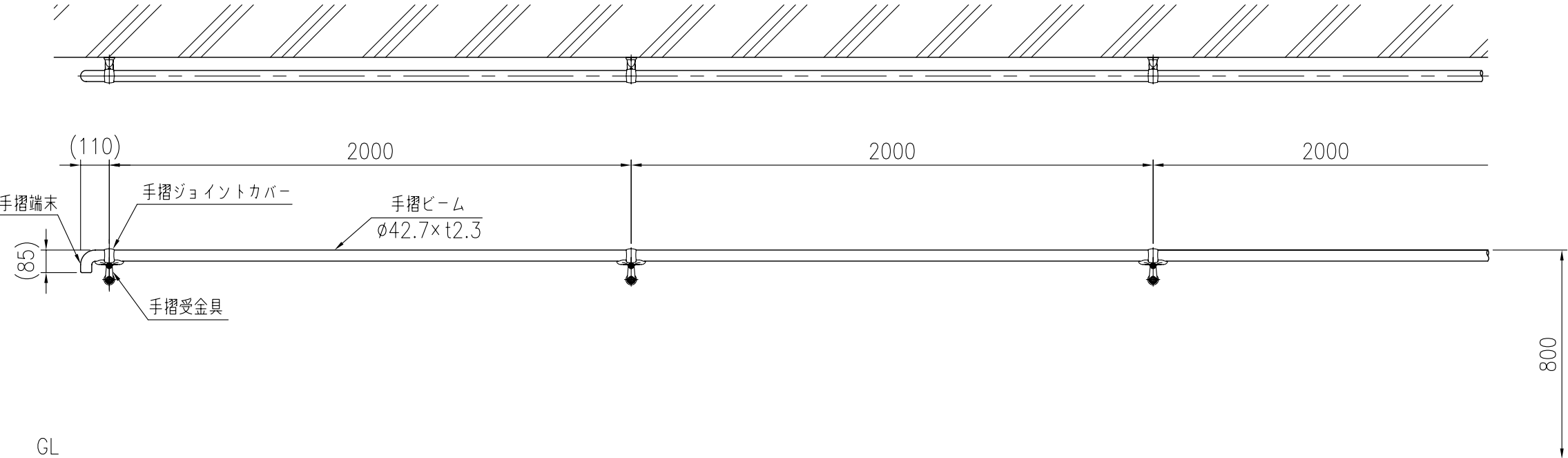
設置図 (1/20)
