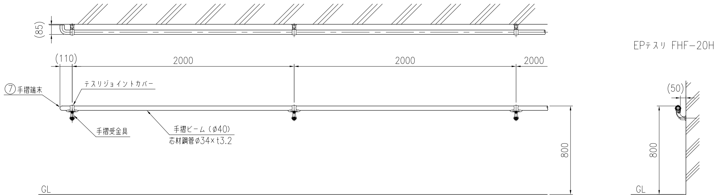
設置図 (1/20)
