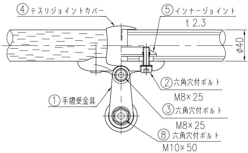
取付部詳細図 (1/3)
