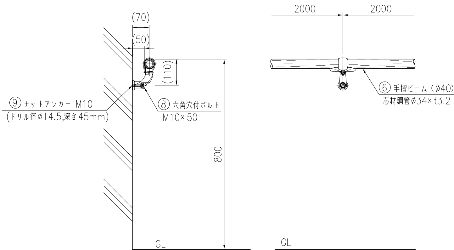
取付図 (1/10)
