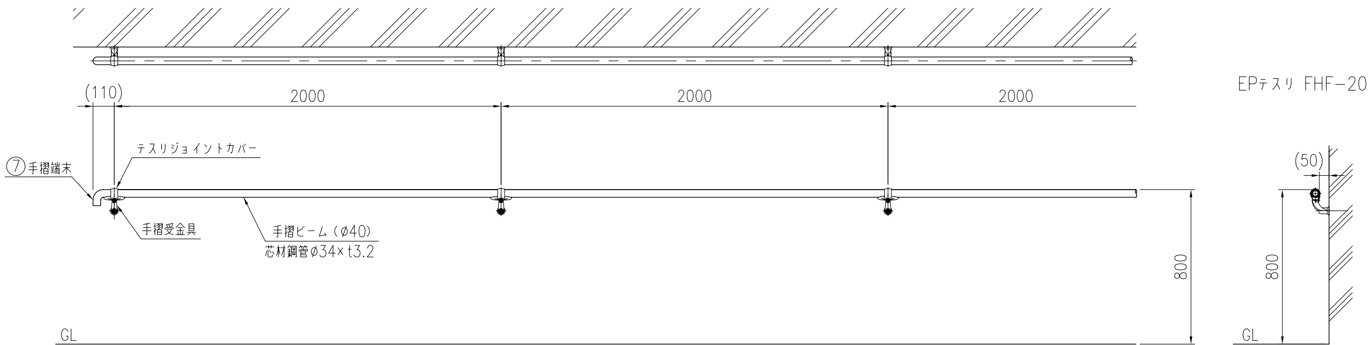
設置図 (1/20)
