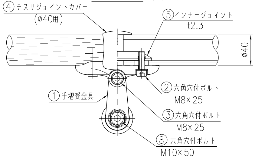
取付部詳細図 (1/3)
