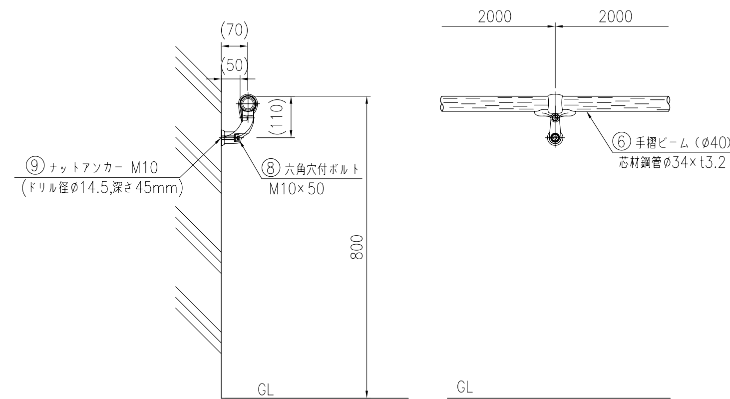
取付図 (1/10)
