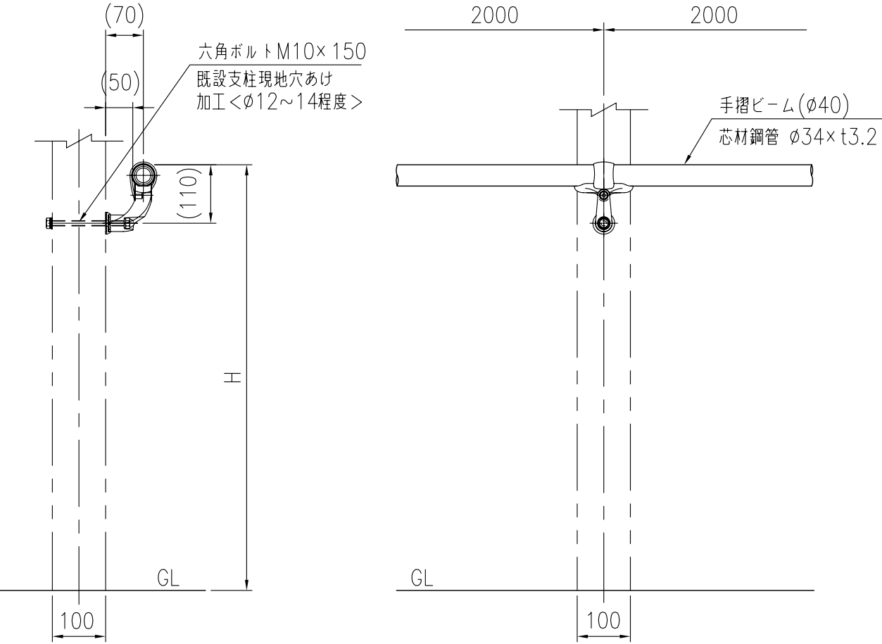
取付図 (1/10)
