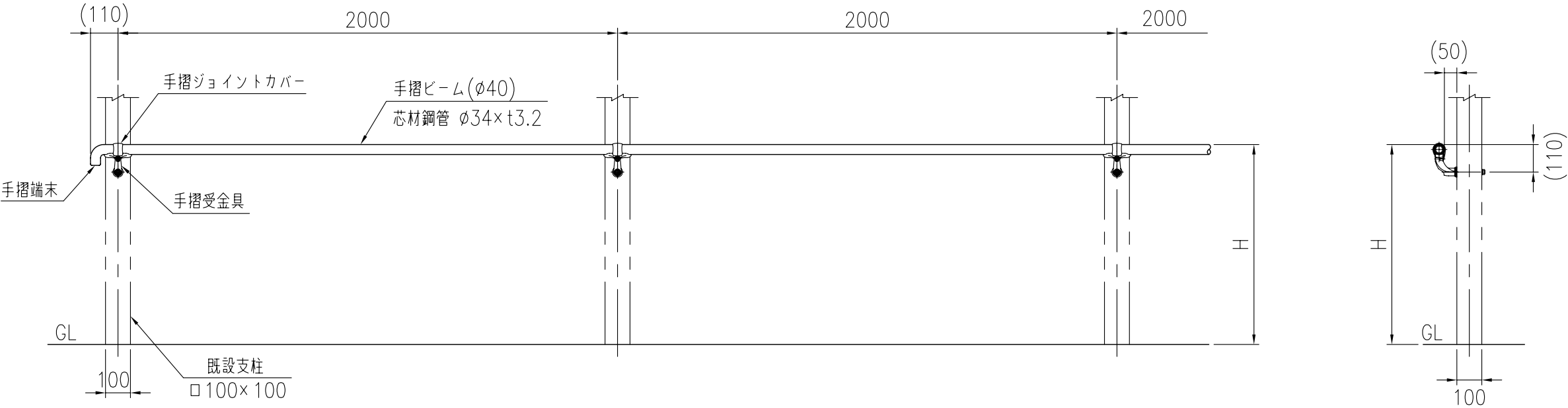
設置図 (1/20)
