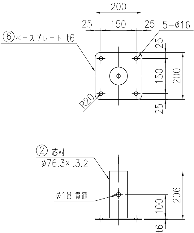
ベースプレート詳細図
