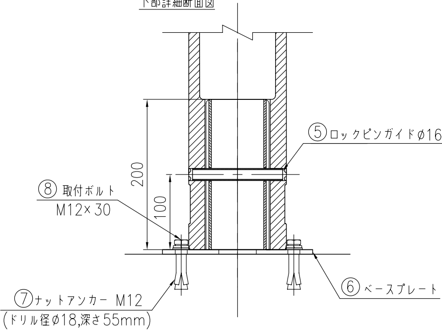
下部詳細断面図
