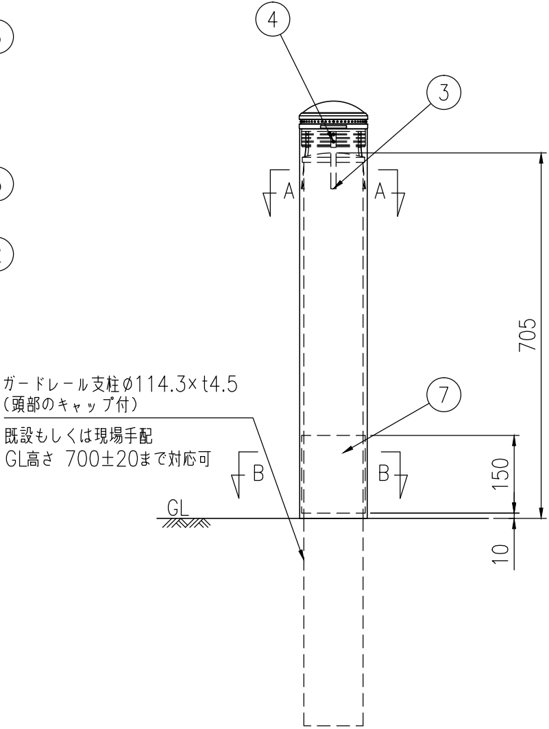
設置図 (1/10)
