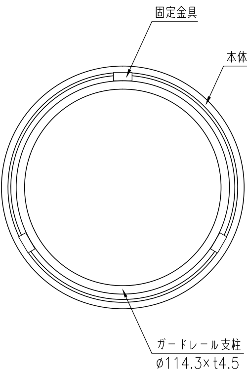
A-A 矢視図 (1/2)
