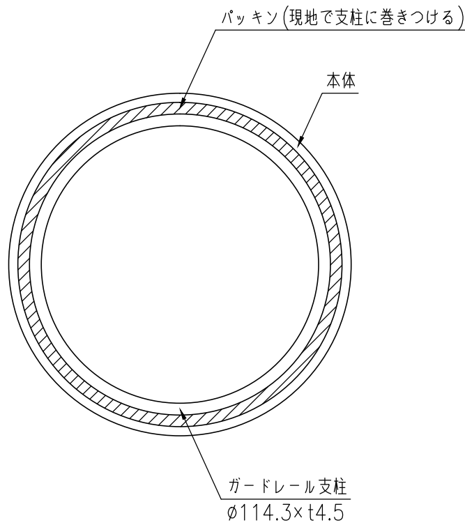
B-B 矢視図 (1/2)
