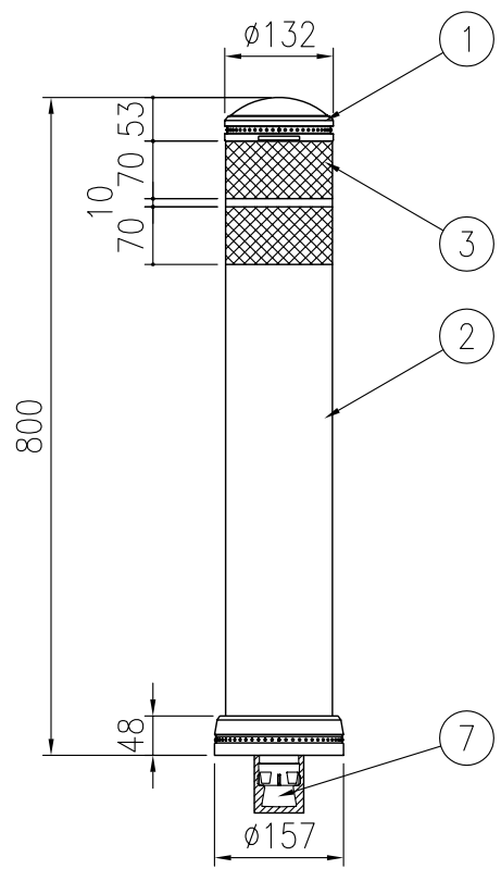
設置図 (1/10)
