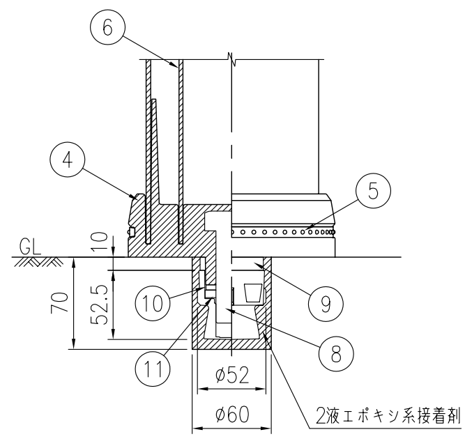
ベース部(設置図) (1/4)
