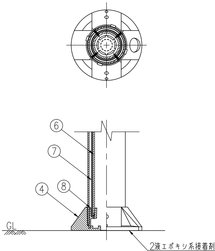
ベース部(設置図) (1/5)
