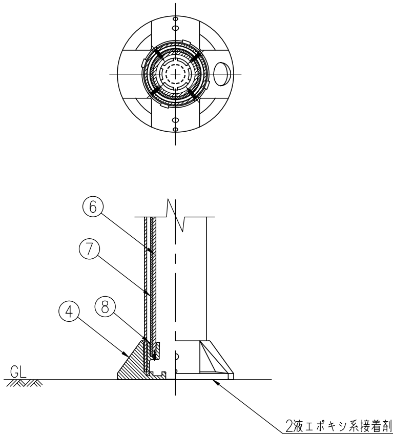
ベース部(設置図) (1/5)
