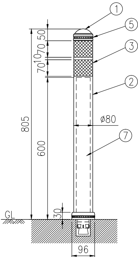
設置図 (1/10)
