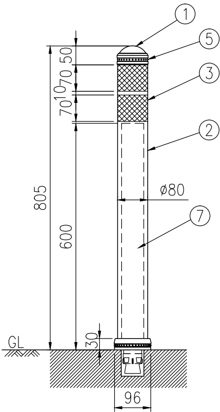
設置図 (1/10)
