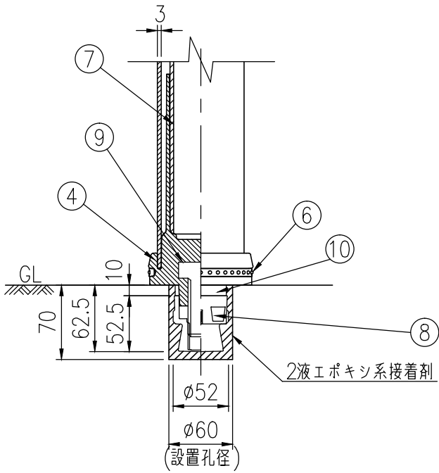
ベース部(設置図) (1/5)
