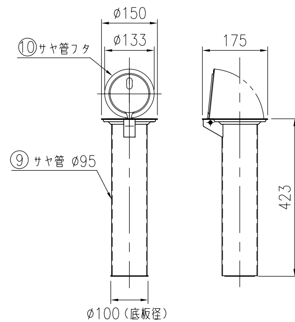
サヤ管詳細図 (1/10)
