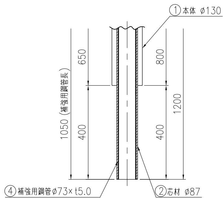
本体下部断面詳細図 (1/10)
