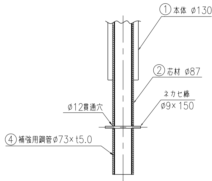
本体下部断面詳細図 (1/10)
