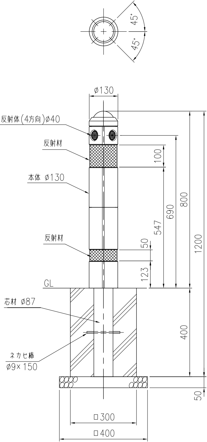
設置図 (1/10)
