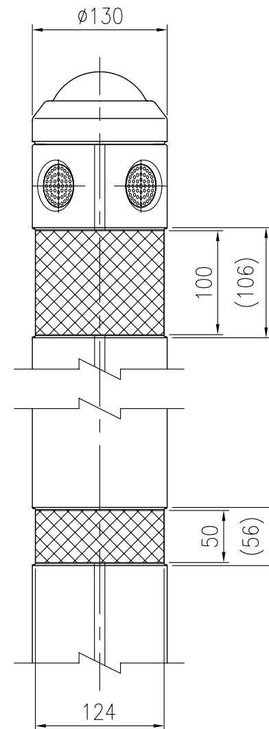
反射材貼付部詳細図 (1/5)
