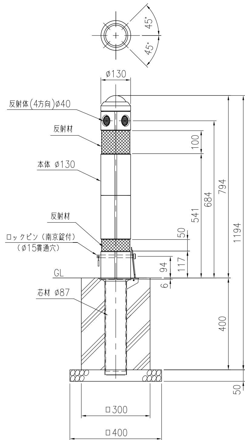
設置図 (1/10)
