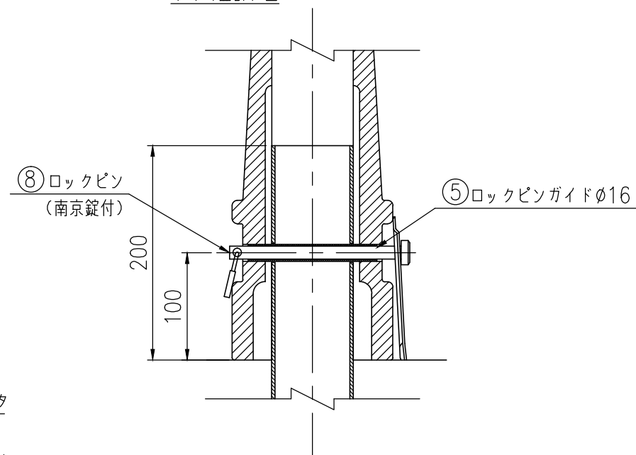
下部断面詳細図
