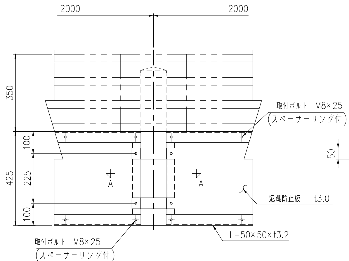
連結部詳細図 (1/10)
