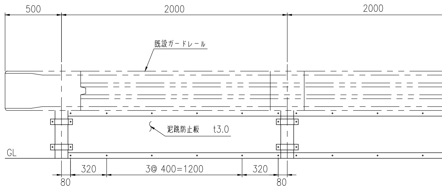
A-A断面詳細図 (1/3)
