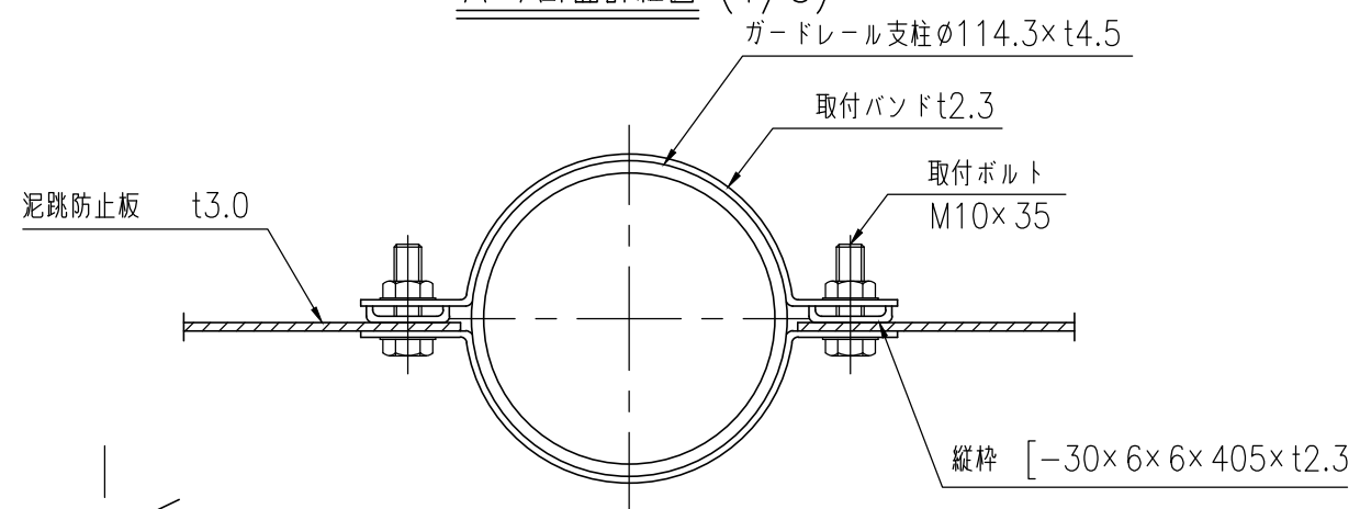
A-A断面詳細図 (1/3)
