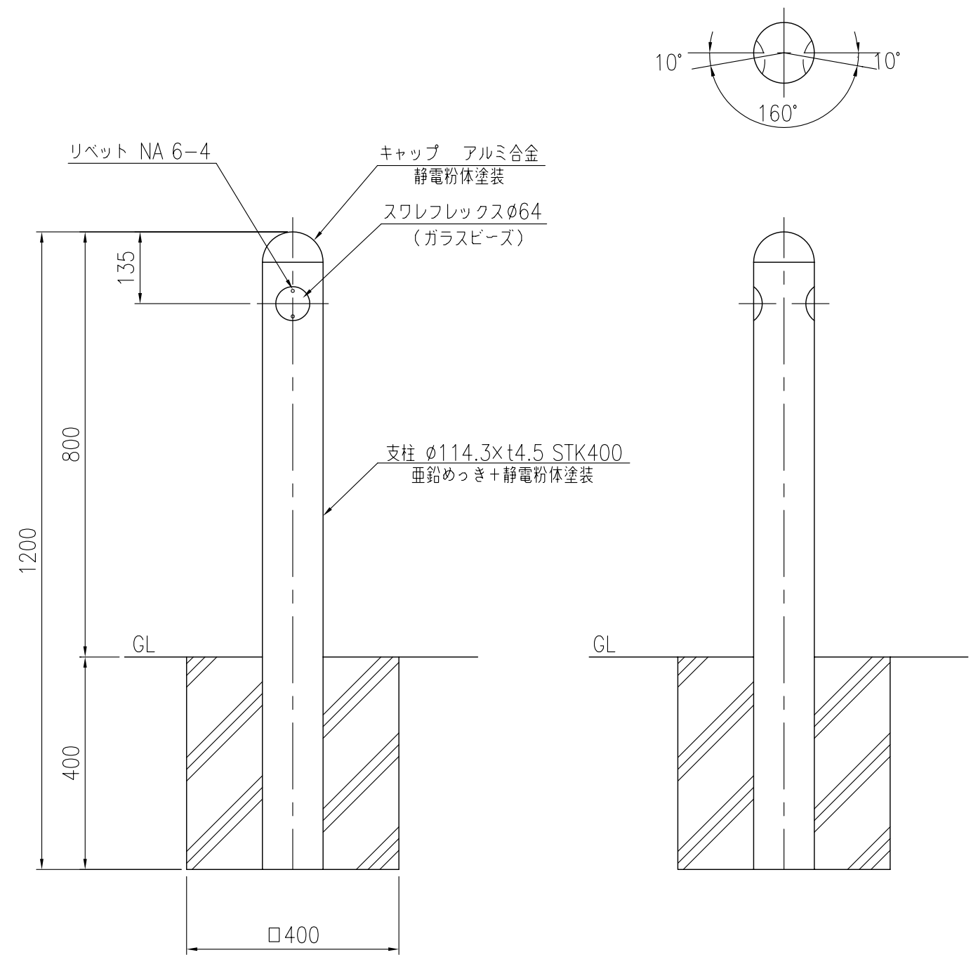
車止め CS6-114-80W
