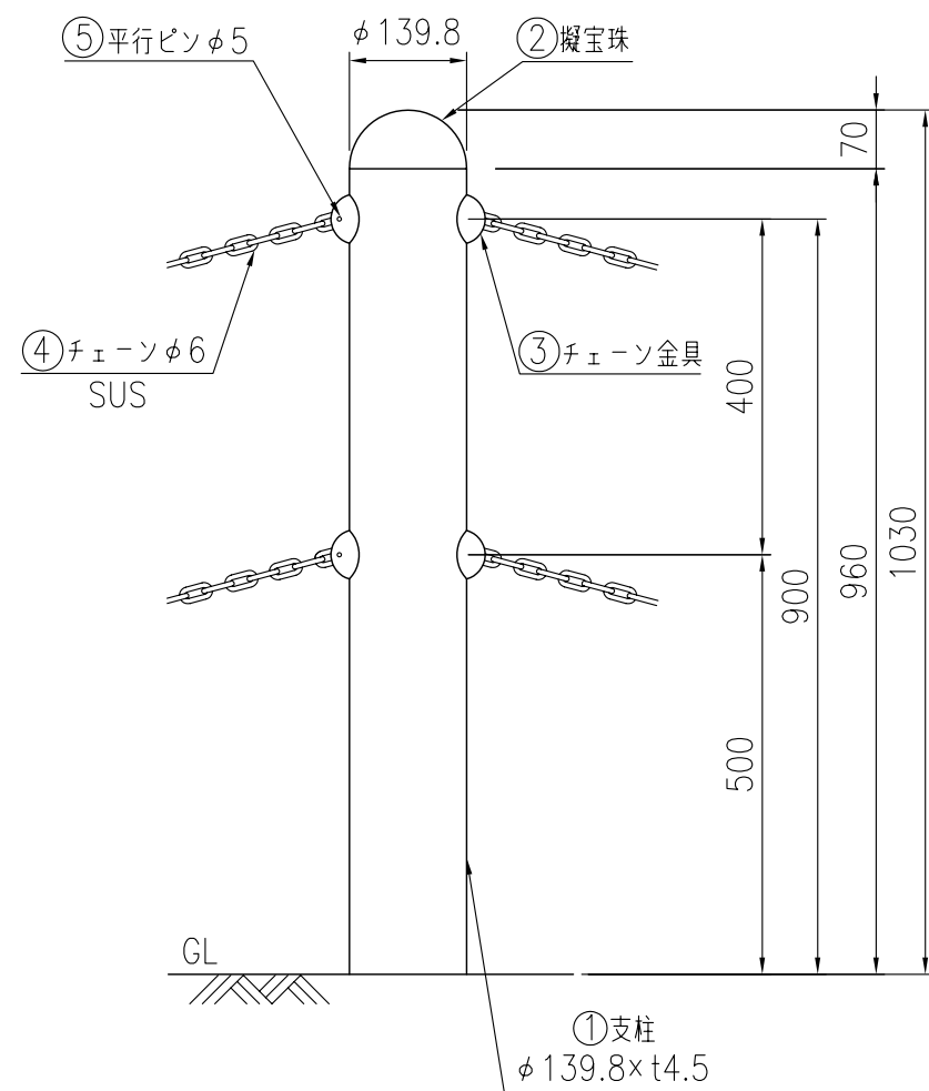
支柱図
