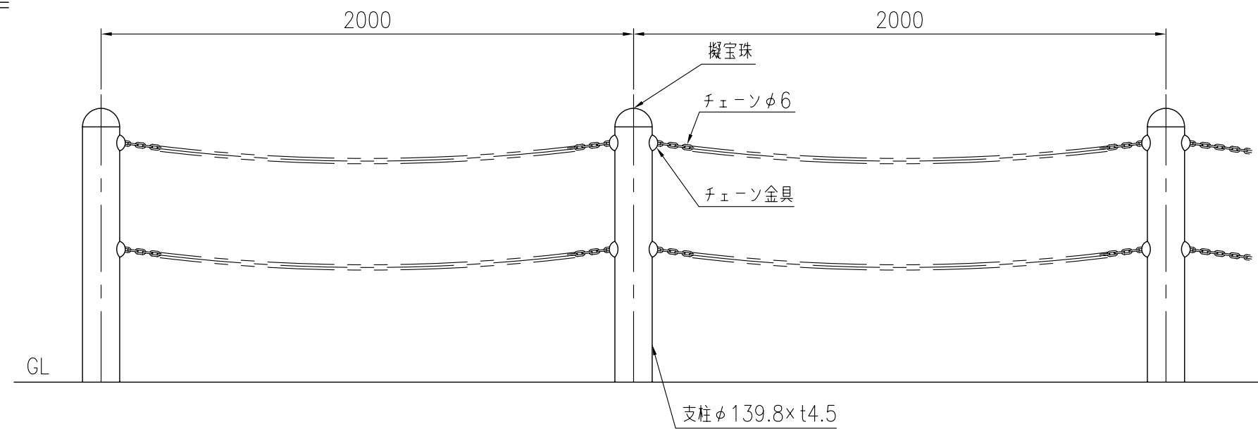
支柱図
