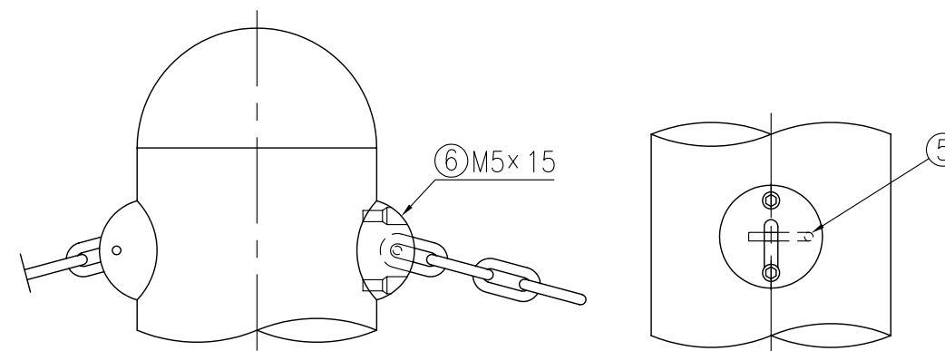
取付部詳細図
