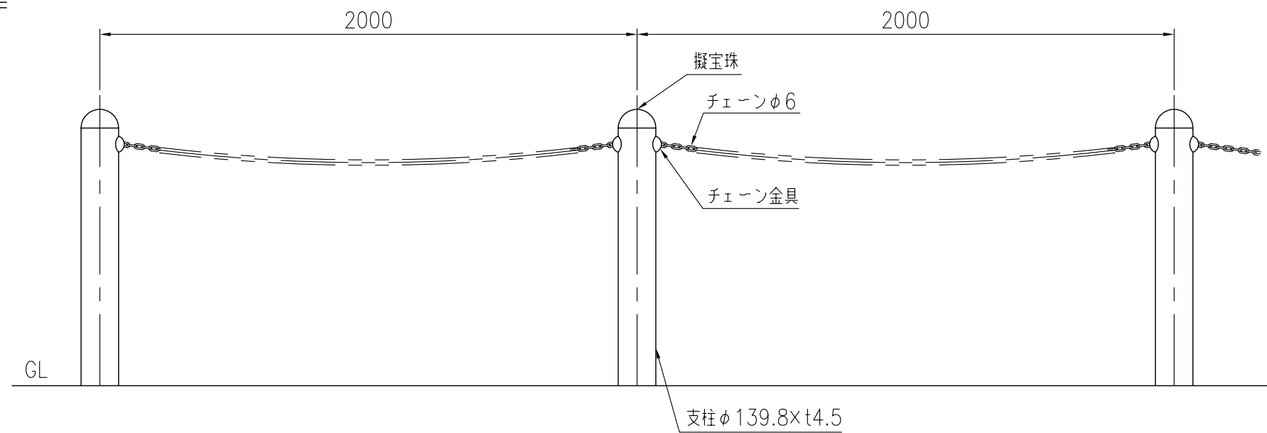
支柱図
