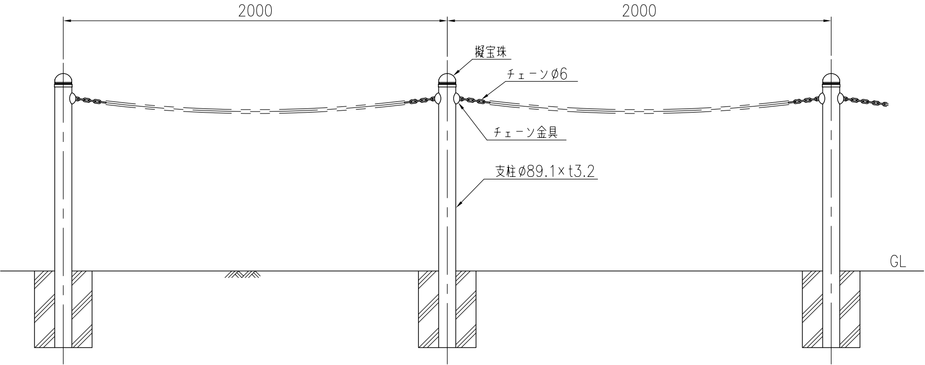
設置図 (1/20)
