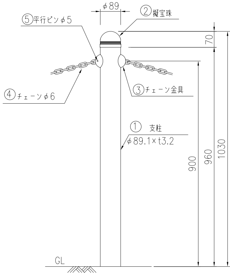
支柱図
