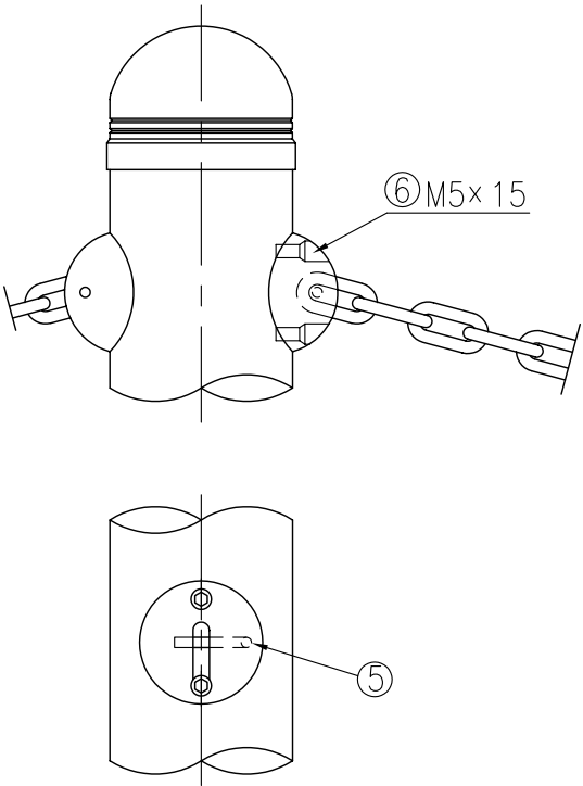
取付部詳細図 (1/4)
