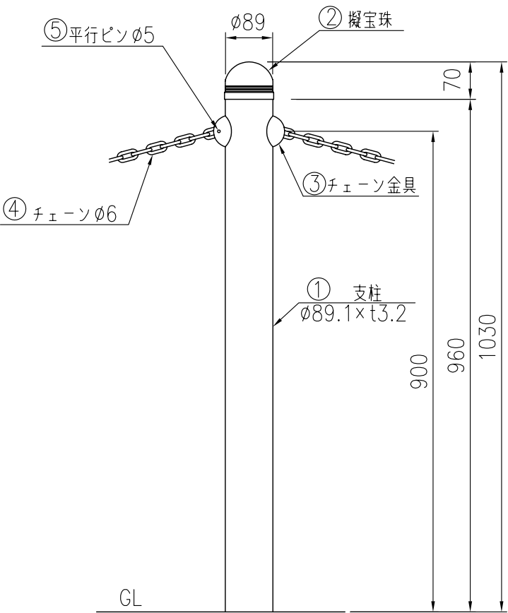
支柱図 (1/10)
