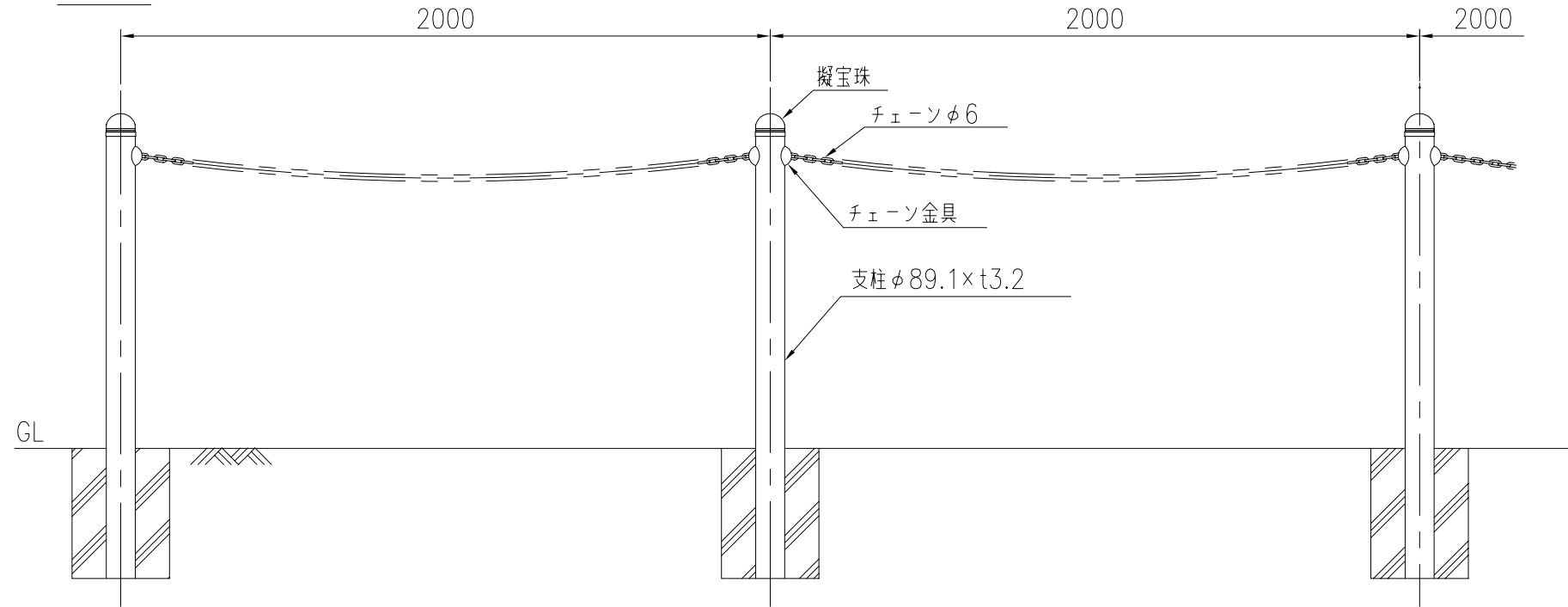
設置図
