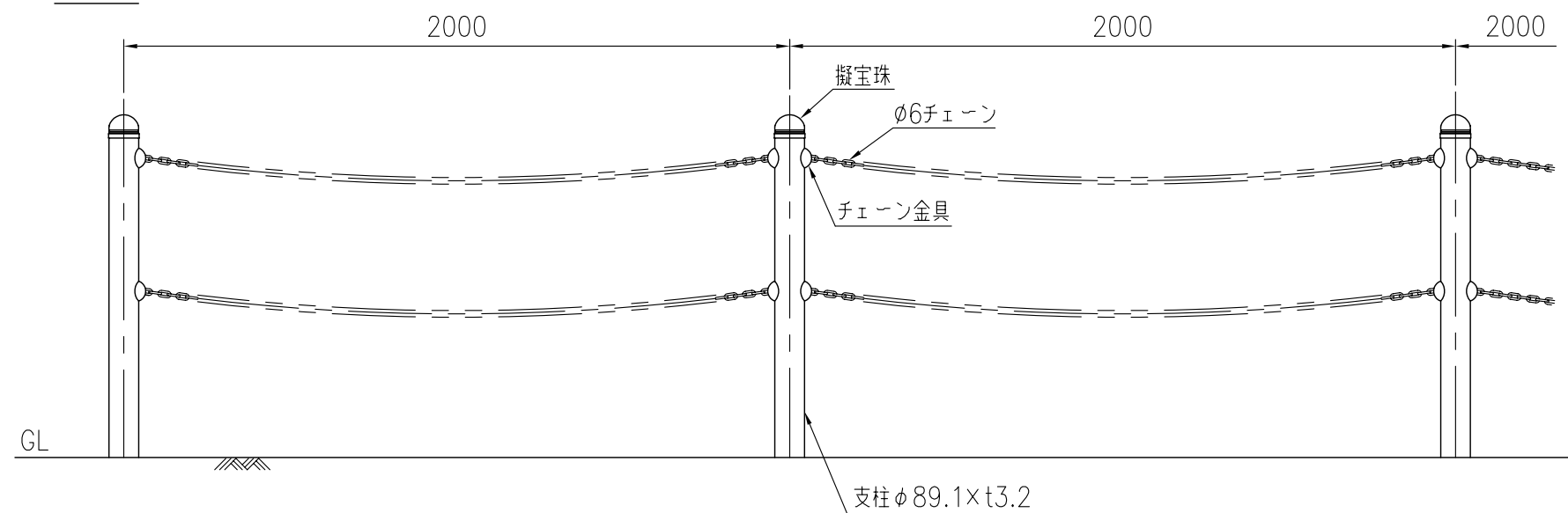
設置図
