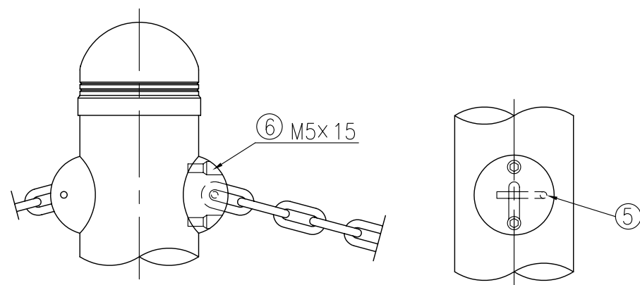
取付詳細図
