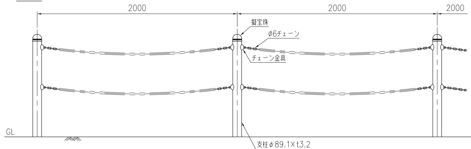
設置図
