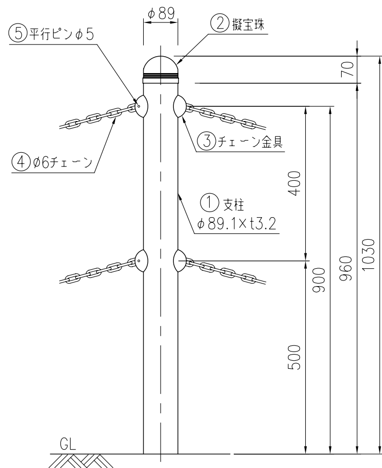
支柱図
