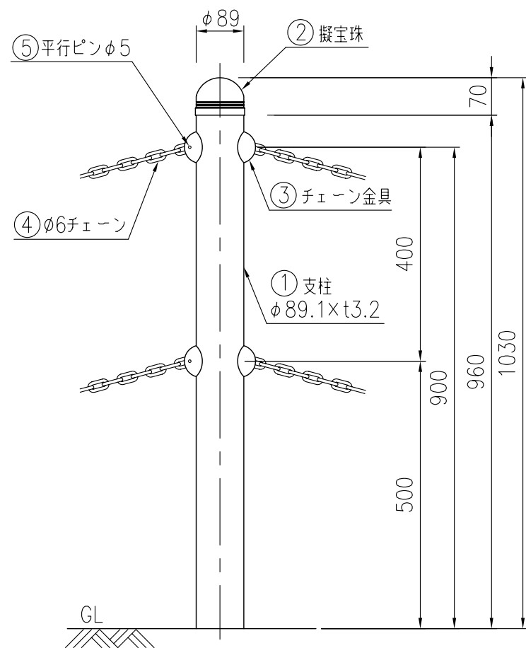
支柱図
