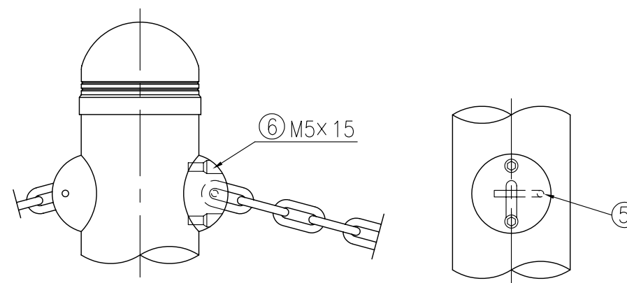
取付詳細図
